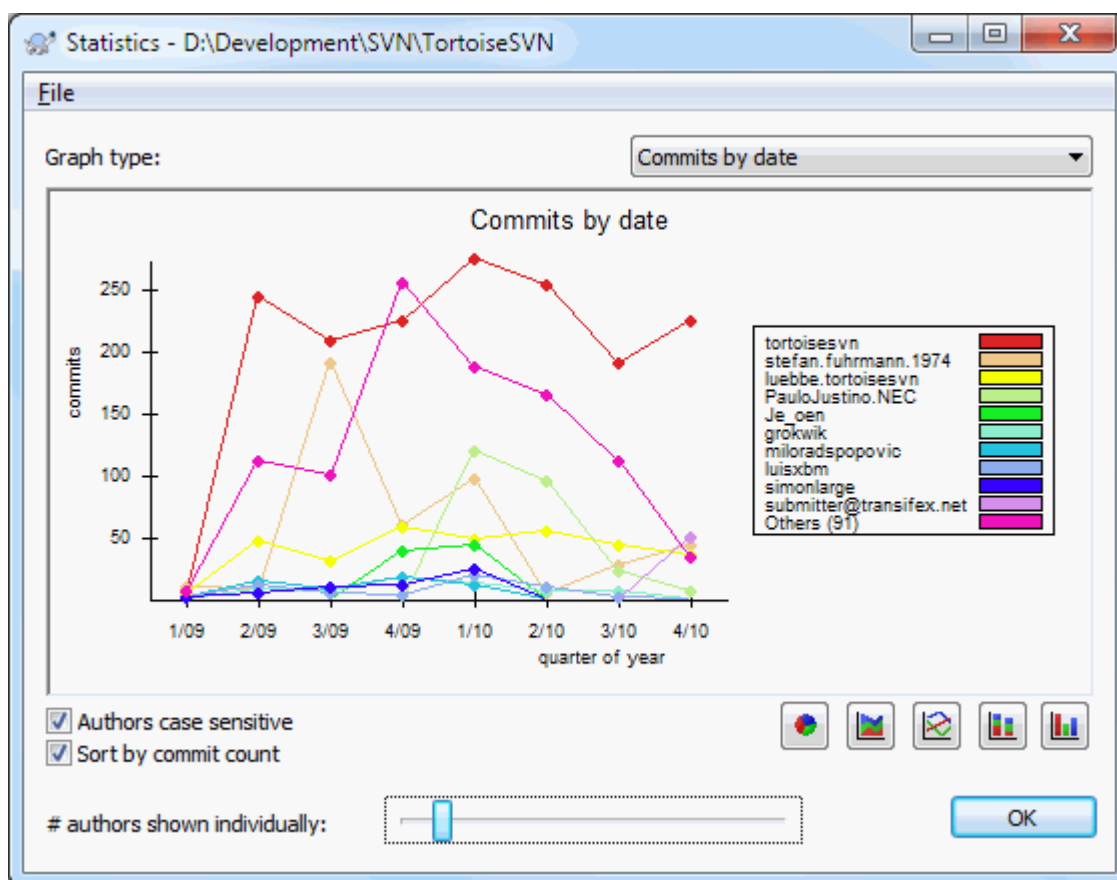
Obrázok 4.25. Commits-by-date Graph
