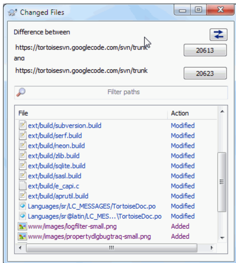
Figure 4.26. La boîte de dialogue Comparer les révisions
