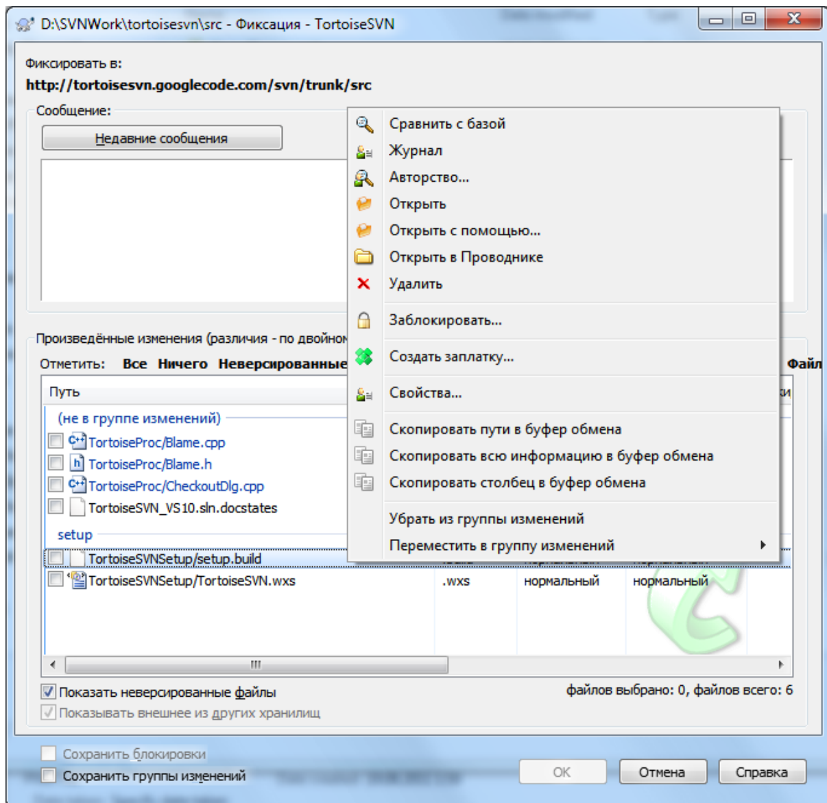
Рисунок 4.8. Диалог фиксации
