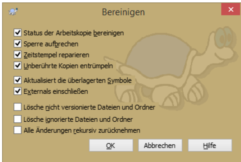
Abbildung 4.34. Der Aufräumen-Dialog
