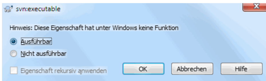
Abbildung 4.47. svn:executable Eigenschaftsseite
