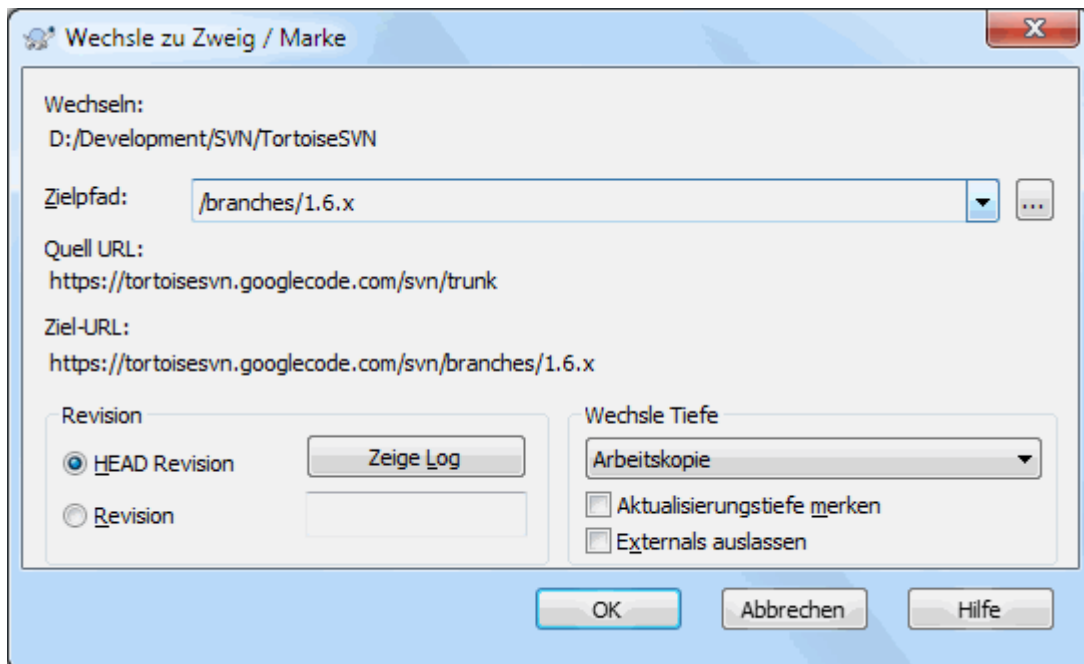
Abbildung 4.50. Der Wechseln-Zu-Dialog
