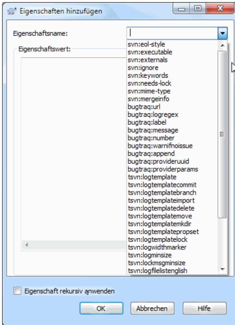
Abbildung 4.36. Eigenschaften hinzufügen
