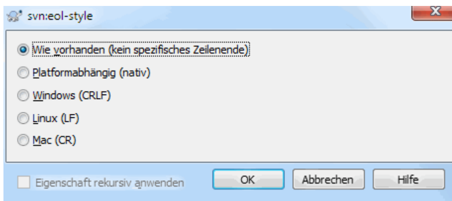
Abbildung 4.41. svn:eol-style Eigenschaftsseite
