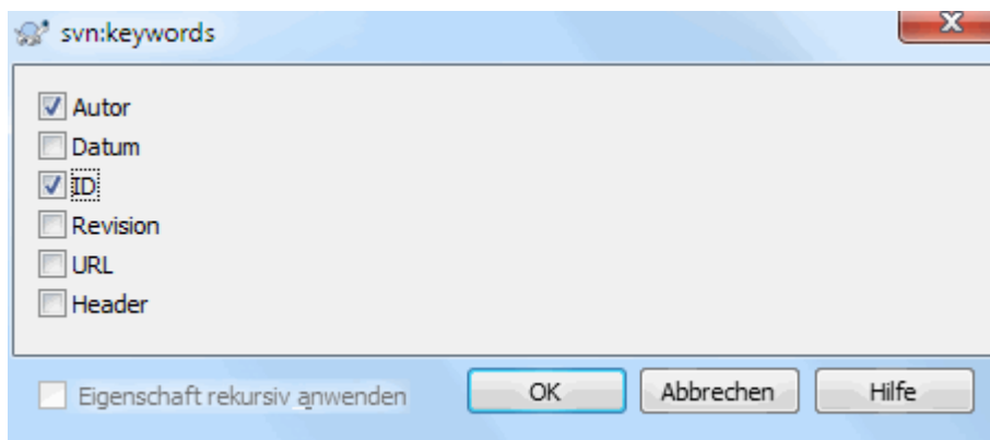
Abbildung 4.40. svn:keywords Eigenschaftsseite
