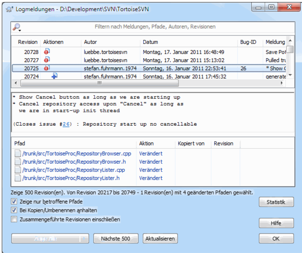
Abbildung 4.16. Der Log-Dialog
