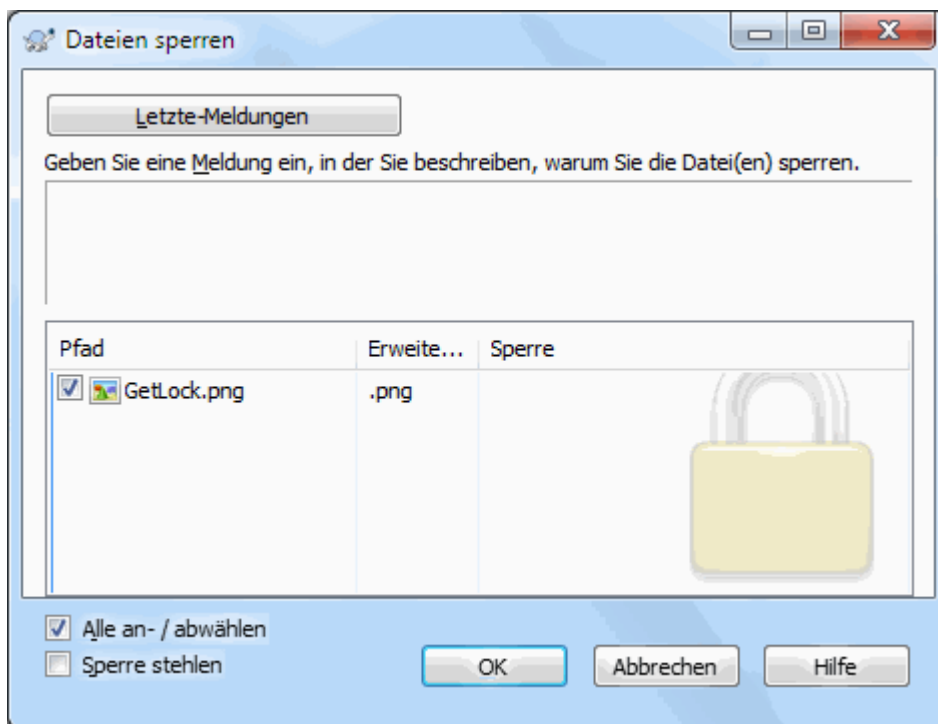
Abbildung 4.55. Der Sperren-Dialog
