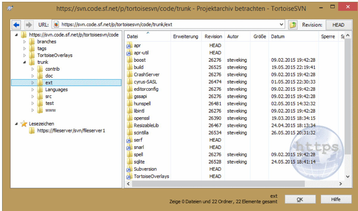
Abbildung 4.60. Projektarchivbetrachter
