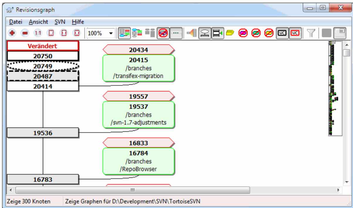
Abbildung 4.61. Ein Revisionsgraph
