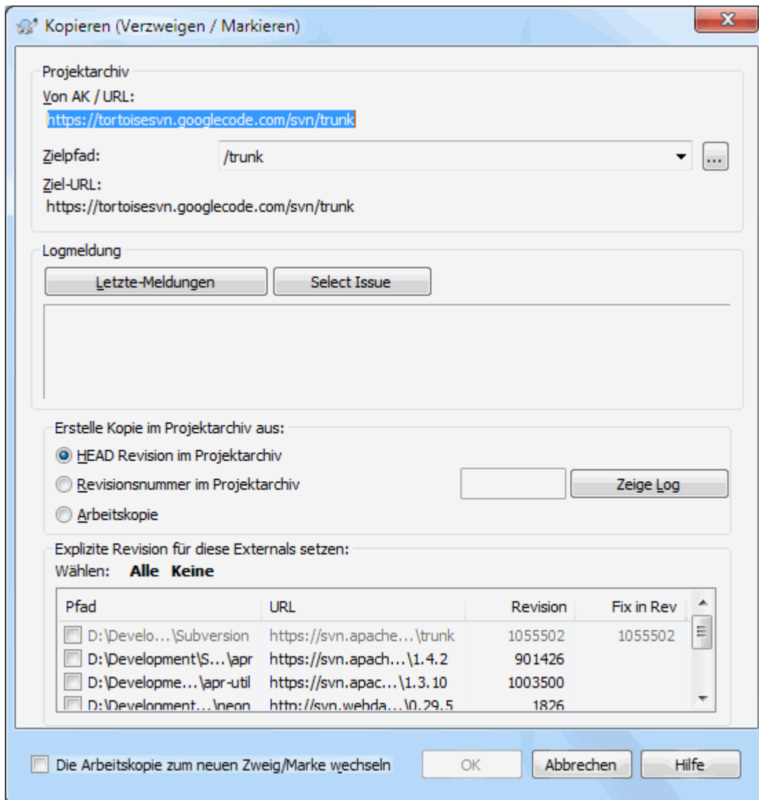
Abbildung 4.49. Der Verzweigen/Markieren-Dialog
