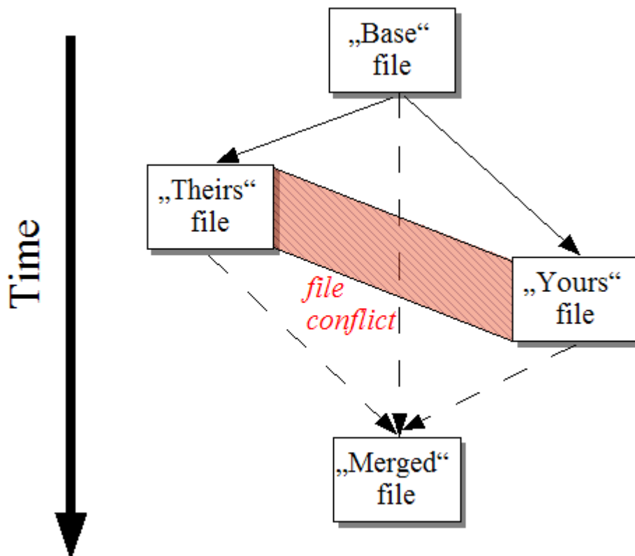
Slika 2.1. Fajl konflikt
