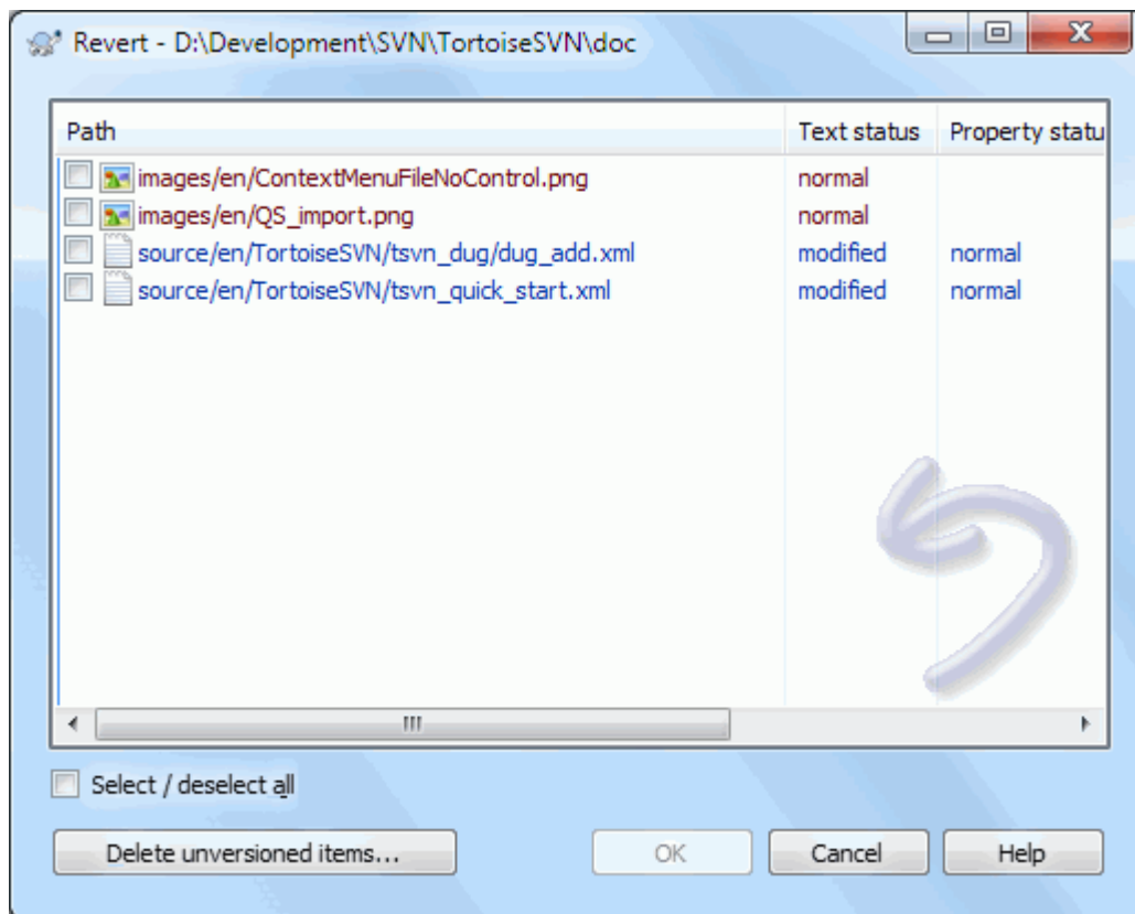
图 4. 32. 恢复对话框
