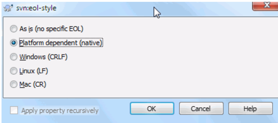
图 4.43. svn:eol-style 属性页
