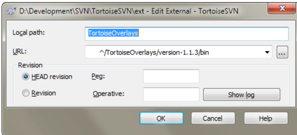
图 4.41. svn:externals 属性页
