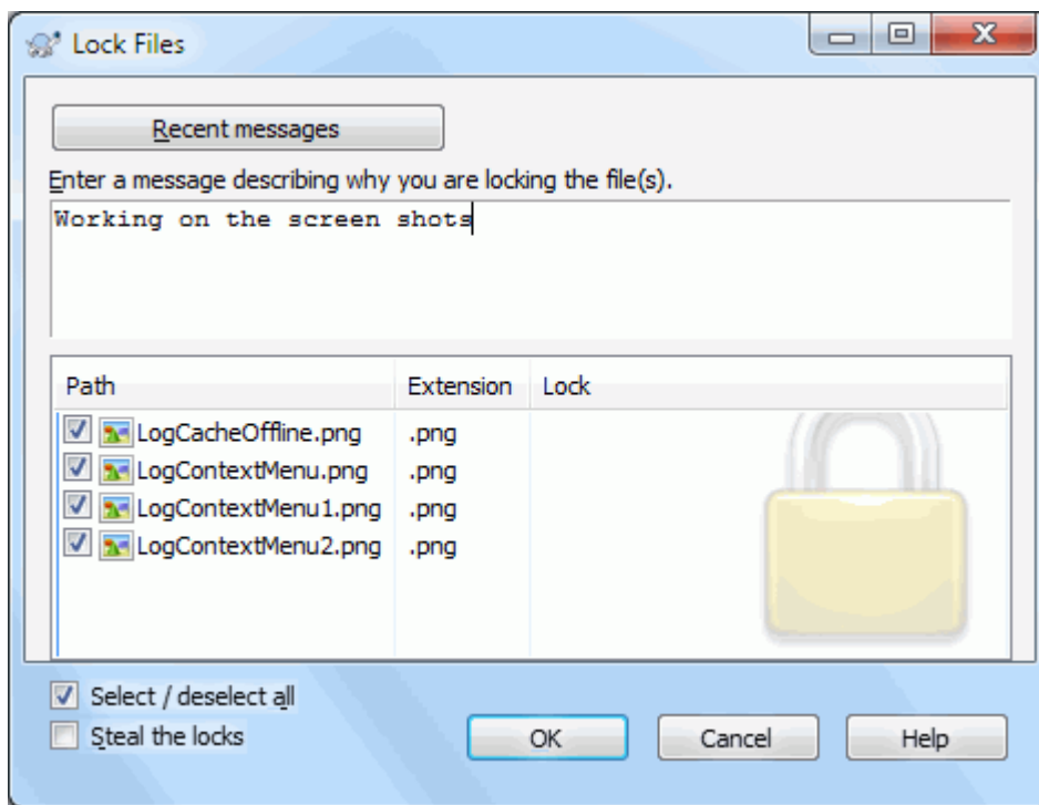
图 4.57. 锁定对话框
