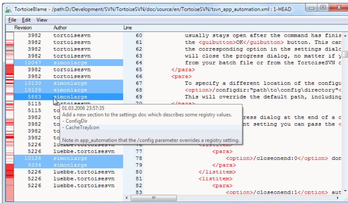
Slika 4.62. TortoiseBlame
