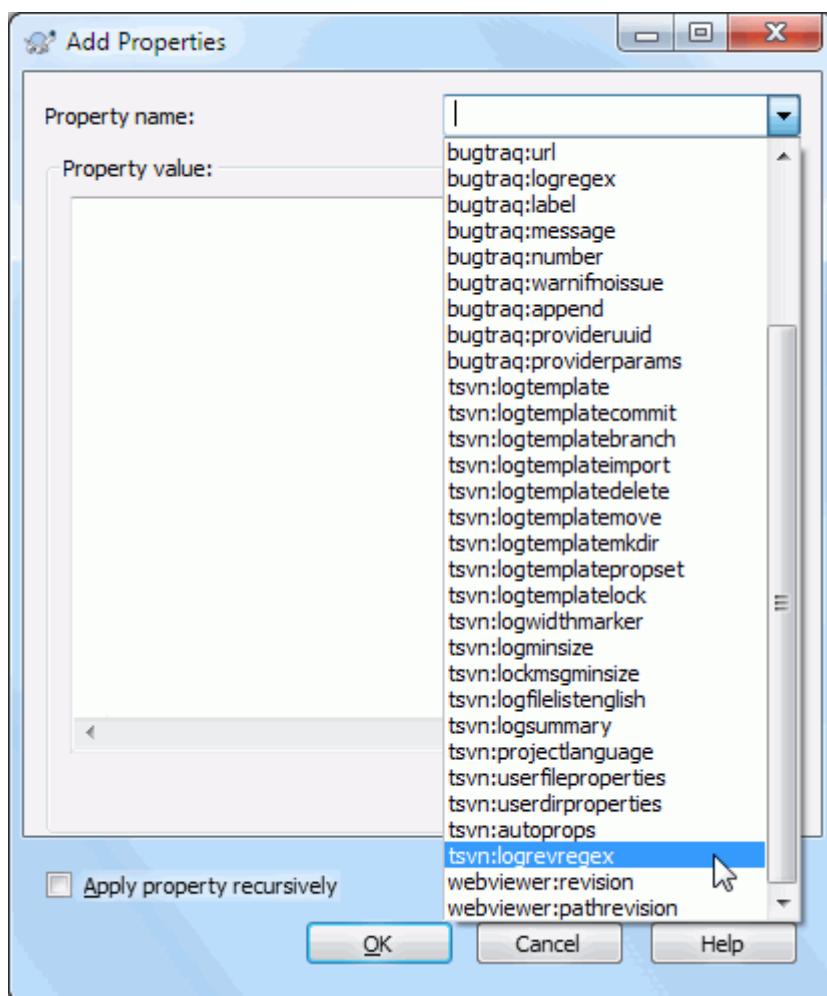
Slika 4.36. Dodajanje lastnosti
