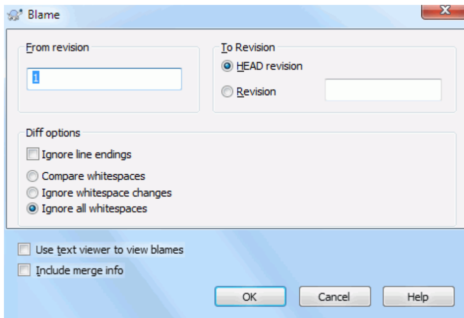
Slika 4.61. Okno hvali/okrivi
