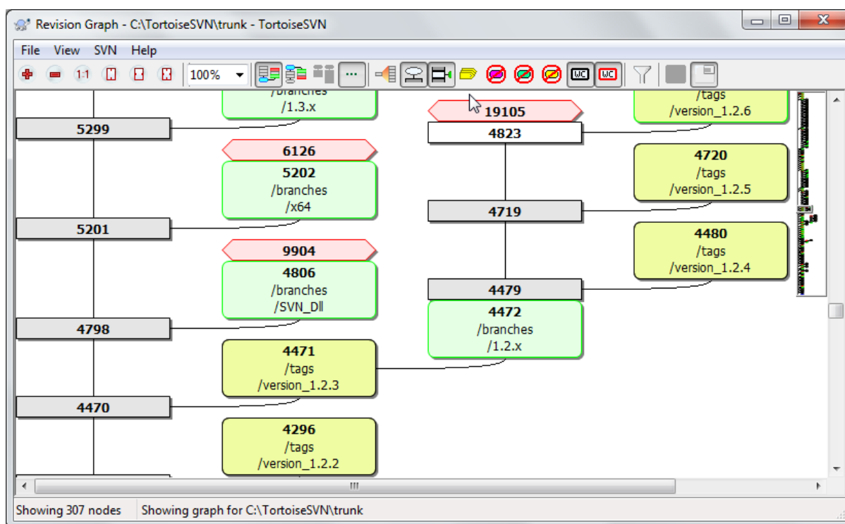
Slika 4.64. Graf revizije
