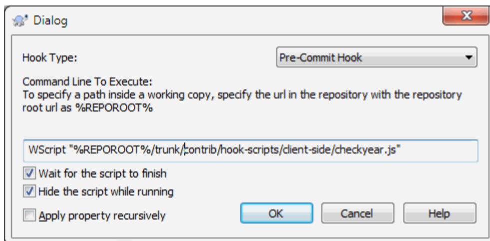
Slika 4.37. Property dialog for hook scripts
