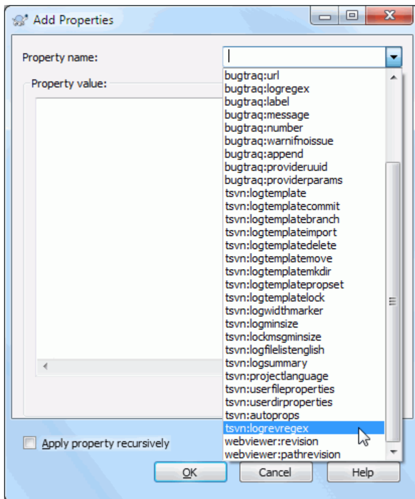
Obrázok 4.36. Pridanie vlastností
