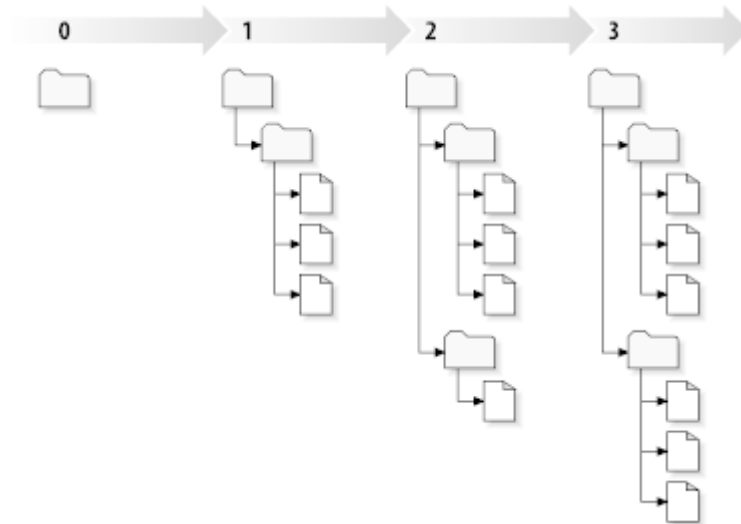
Obrázok 2.7. Úložisko
