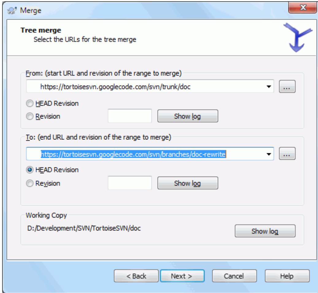
图 4.54. 合并向导 - 树合并
