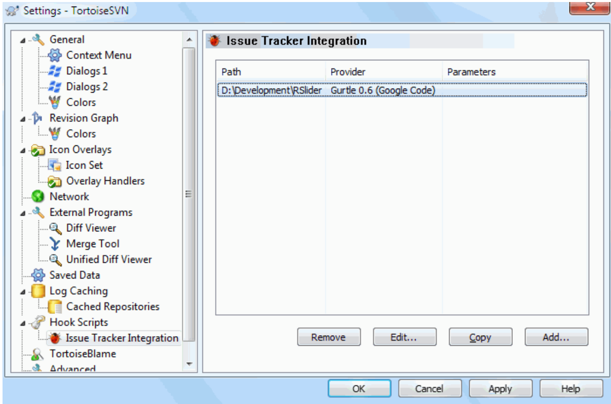
图 4.87. 设置对话框，问题跟踪集成页
