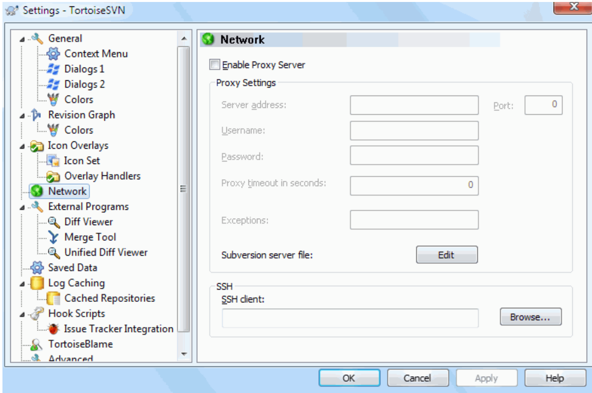
图 4.79. 设置对话框，网络设置页面
