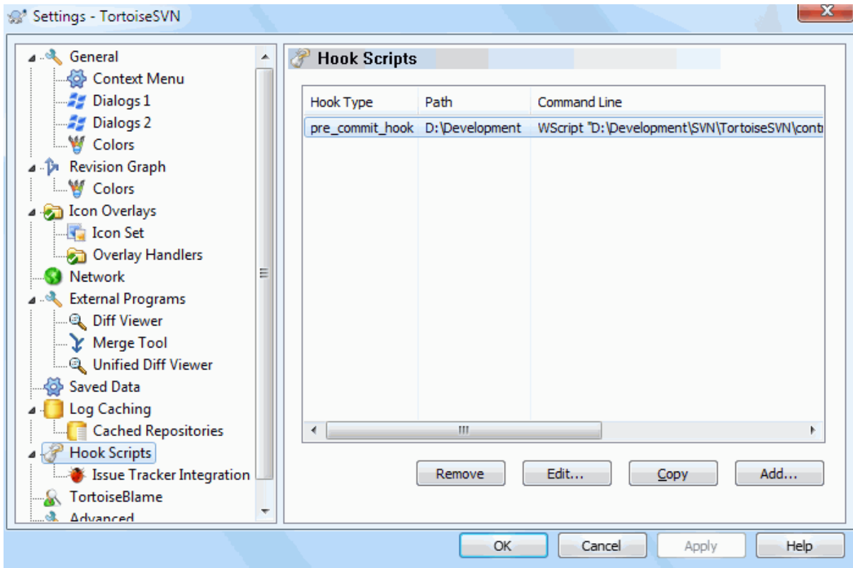
图 4.85. 设置对话框，钩子脚本页
