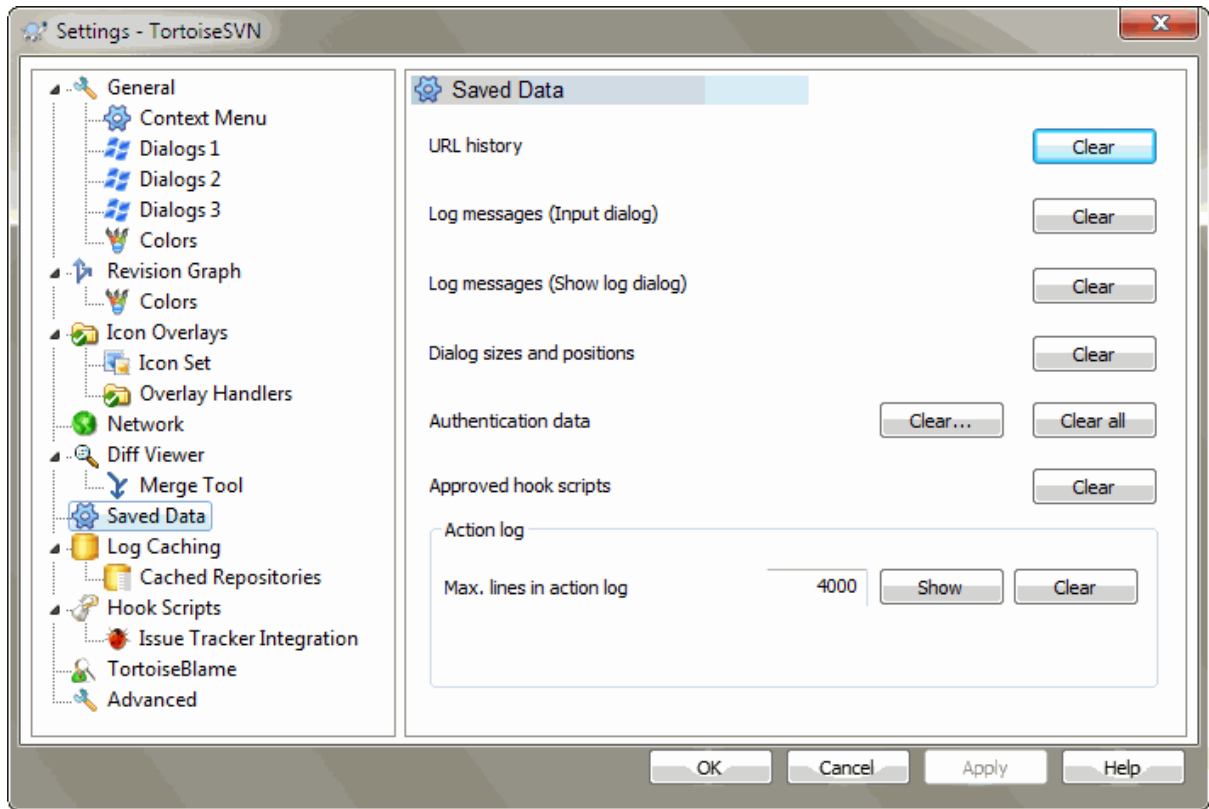
图 4.82. 设置对话框，已保存数据设置页面
