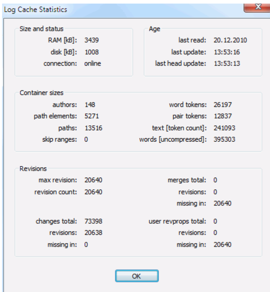
图 4.84. 设置对话框，日志缓存统计
