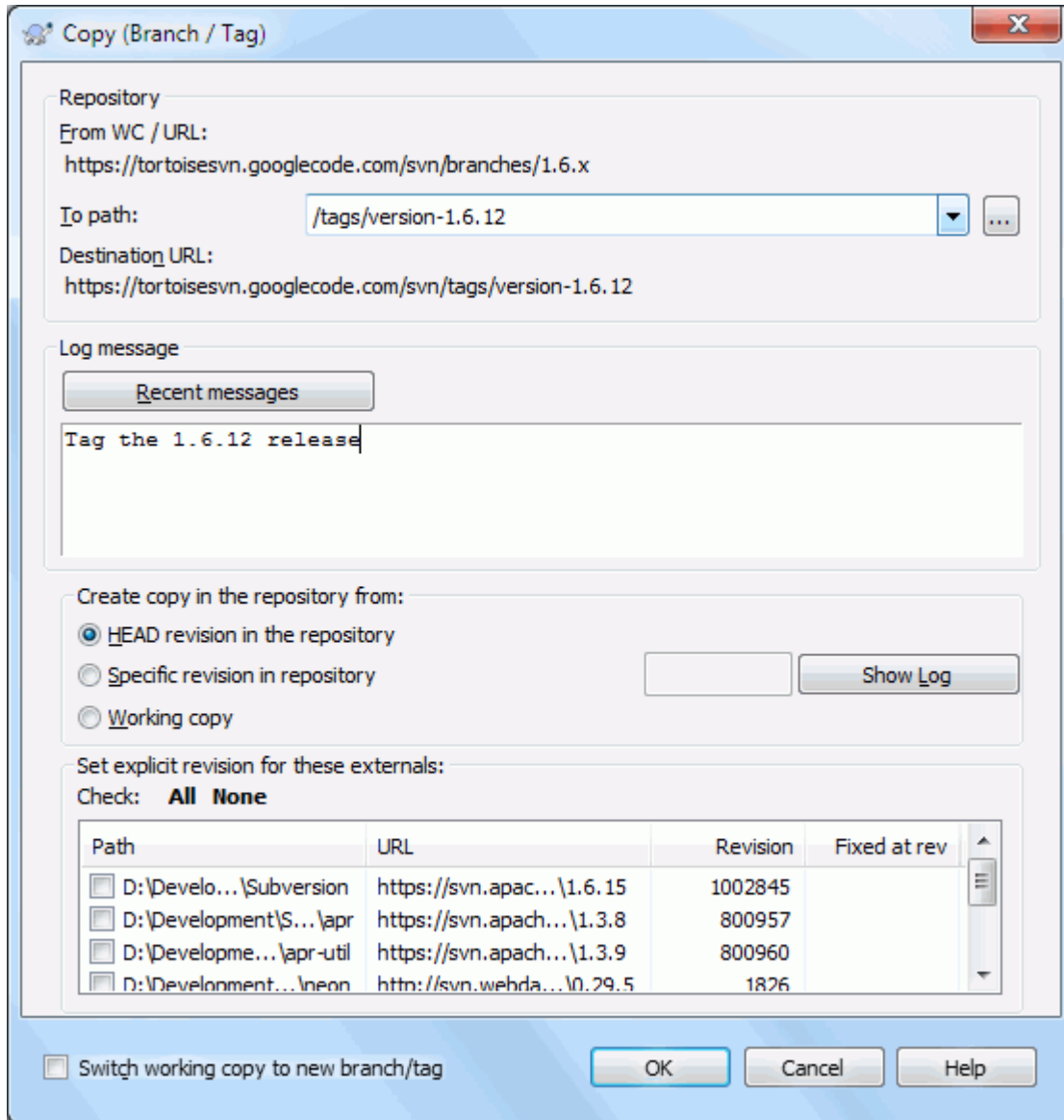
图 4.51. 分支/标记对话框
