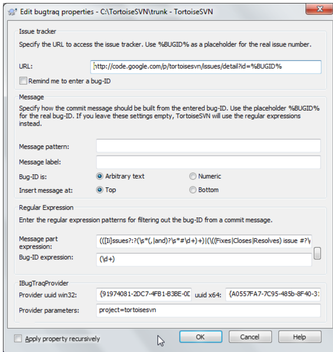
Rysunek 4.67. Okno dialogowe atrybutów bugtraq
