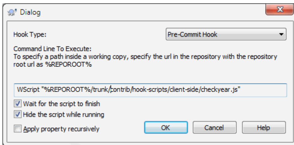
Rysunek 4.37. Okno dialogowe atrybutów skryptów przechwytyjących
