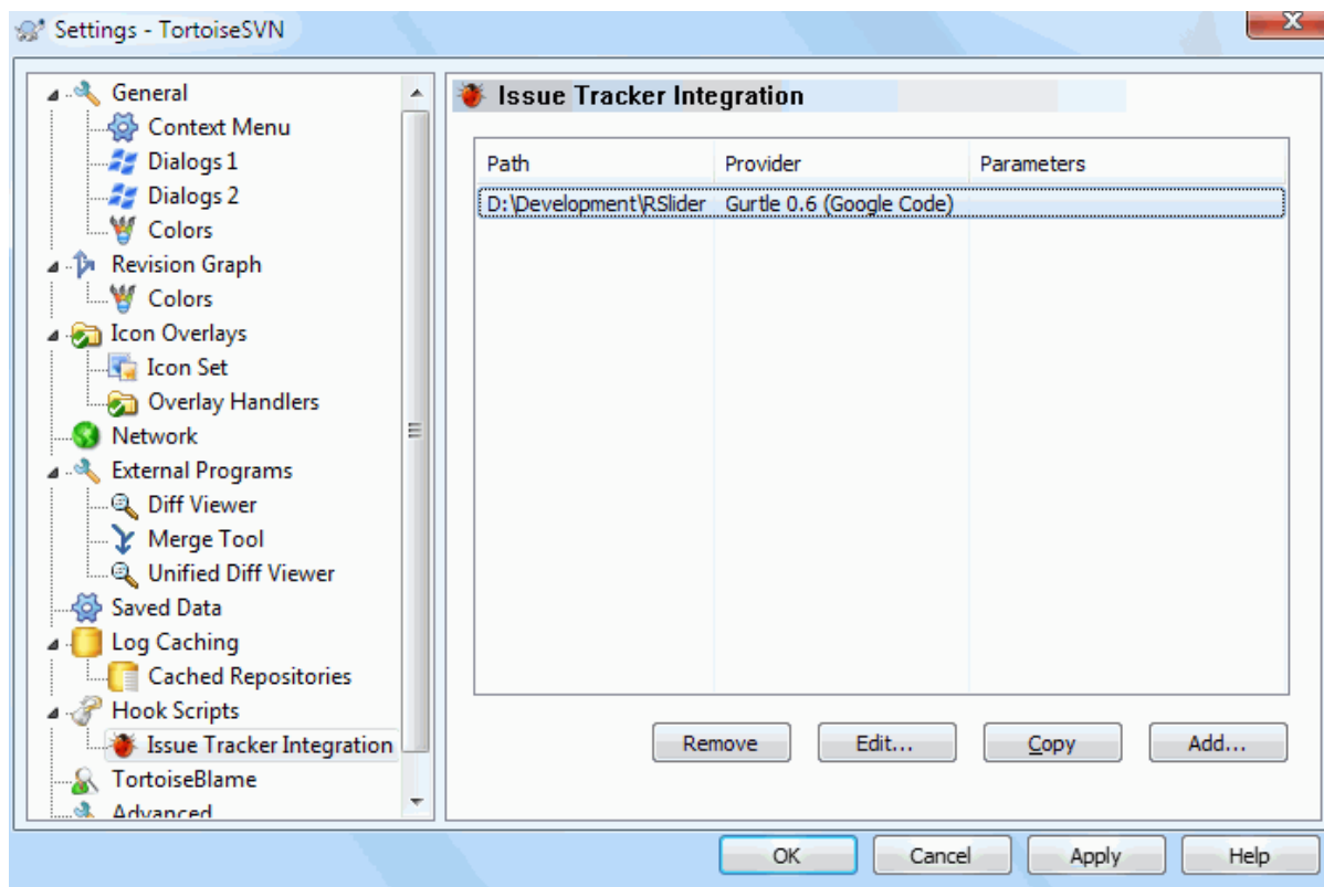
Rysunek 4.88. Okno dialogowe ustawień, strona Integracja z systemami śledzenia błędów
