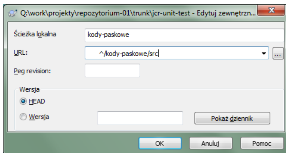
Rysunek 4.42. Strona atrybutu svn:externals
