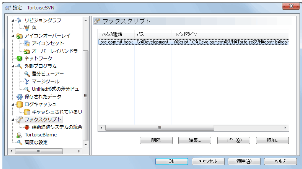
図4. 85 設定ダイアログの「フックスクリプト」ページ
