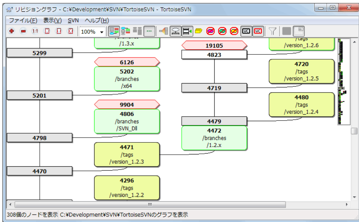
図4.63 リビジョングラフ
