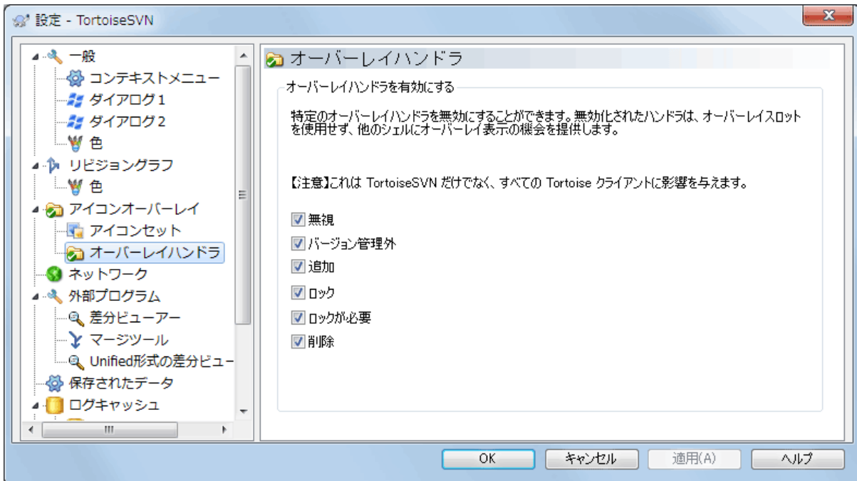
図4.78 設定ダイアログの「オーバーレイハンドラー」ページ
