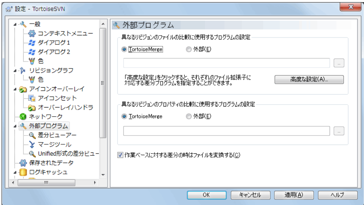
図4. 80 設定ダイアログの「差分ビューアー」ページ
