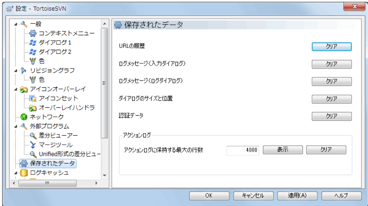
図4. 82 設定ダイアログの「保存されたデータ」ページ
