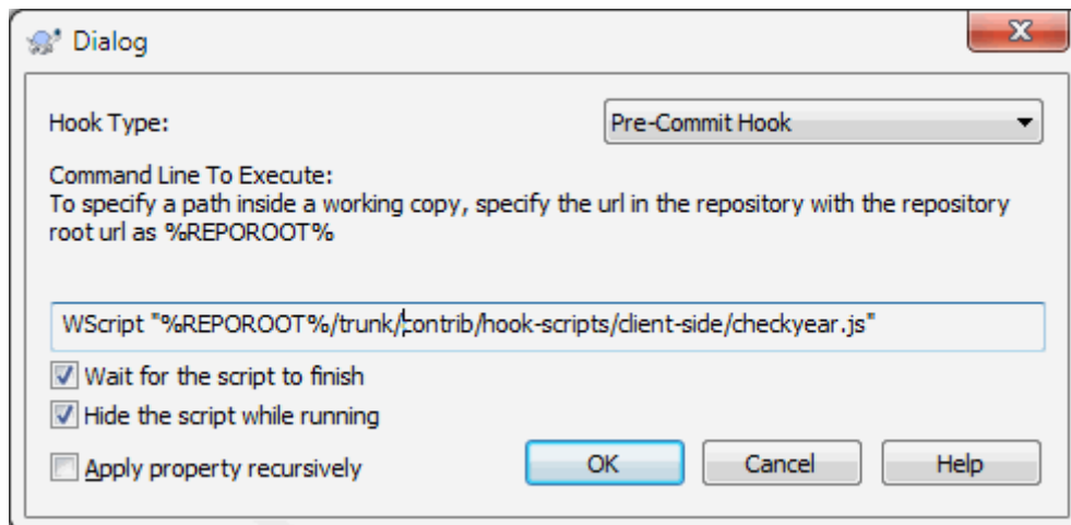
図4.36 フックスクリプトのプロパティダイアログ
