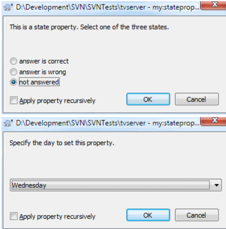
図4.38 state型のユーザープロパティダイアログ
