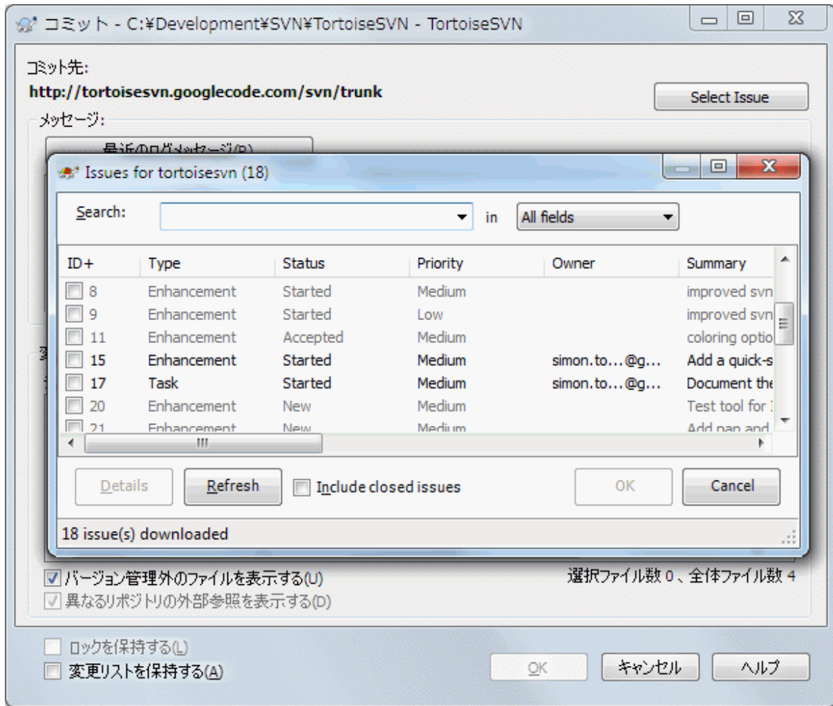
図4.67 課題追跡システムクエリダイアログの例
