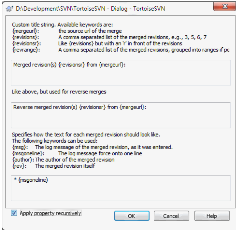
図4.50 プロパティダイアログのマージログメッセージのテンプレート設定
