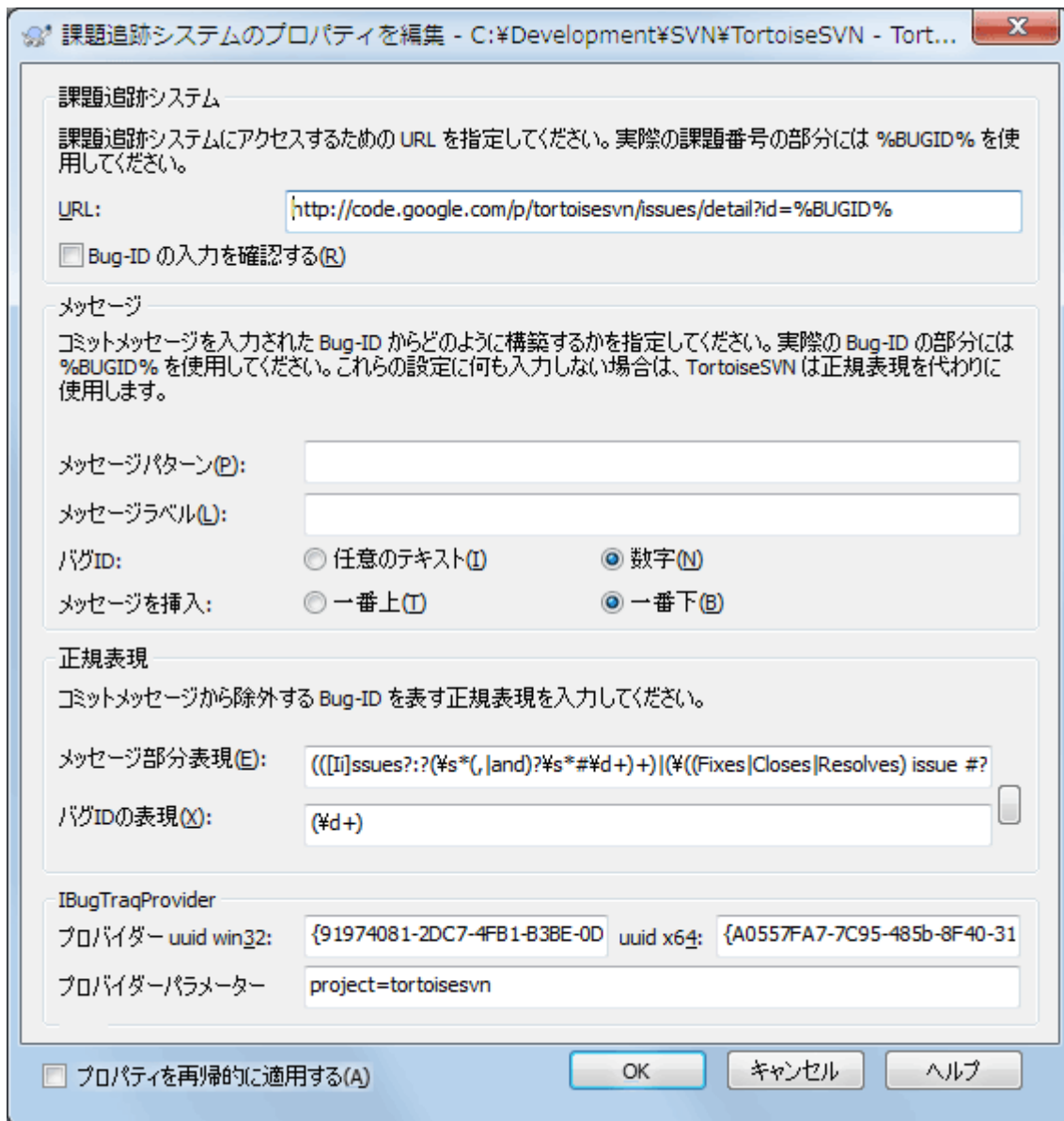
図4.44 tsvn:bugtraq プロパティページ
