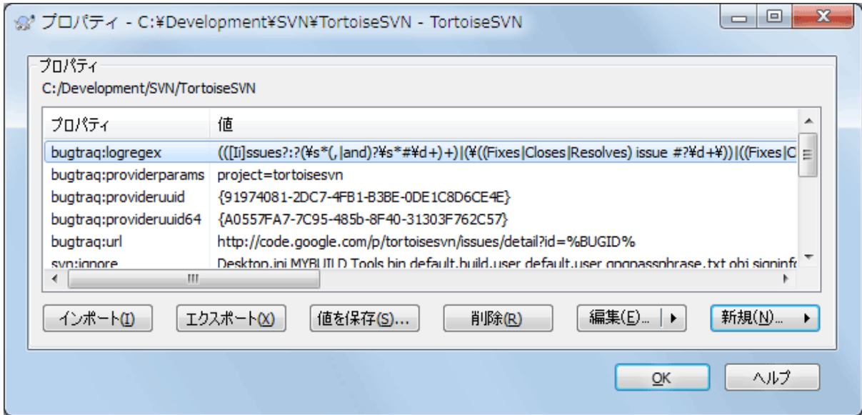
図4.34 Subversion のプロパティページ
