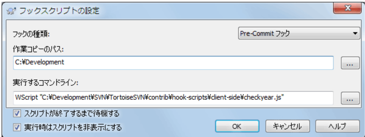
図4. 86 設定ダイアログのフックスクリプトの設定
