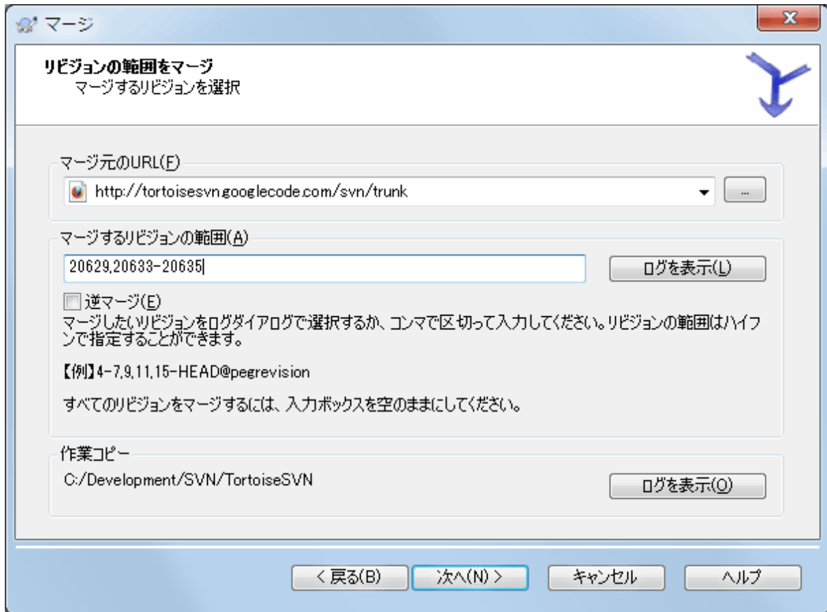
図4.53 マージウィザード - リビジョン範囲の選択
