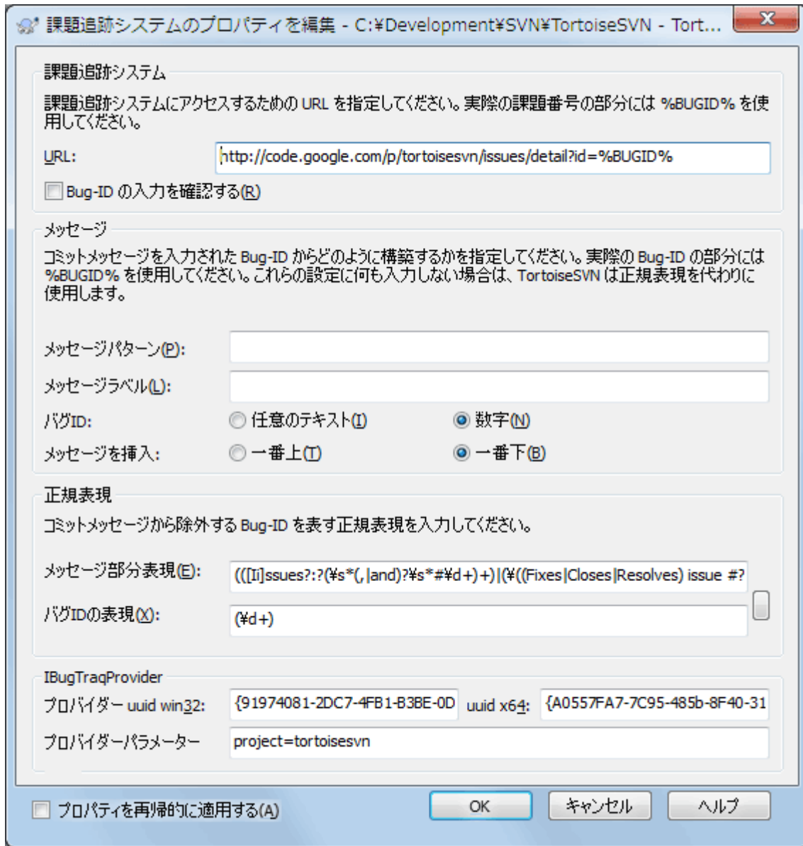
図4. 66 課題追跡システムのプロパティダイアログ
