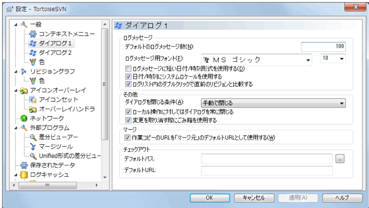
図4.70 設定ダイアログの「ダイアログ 1」ページ
