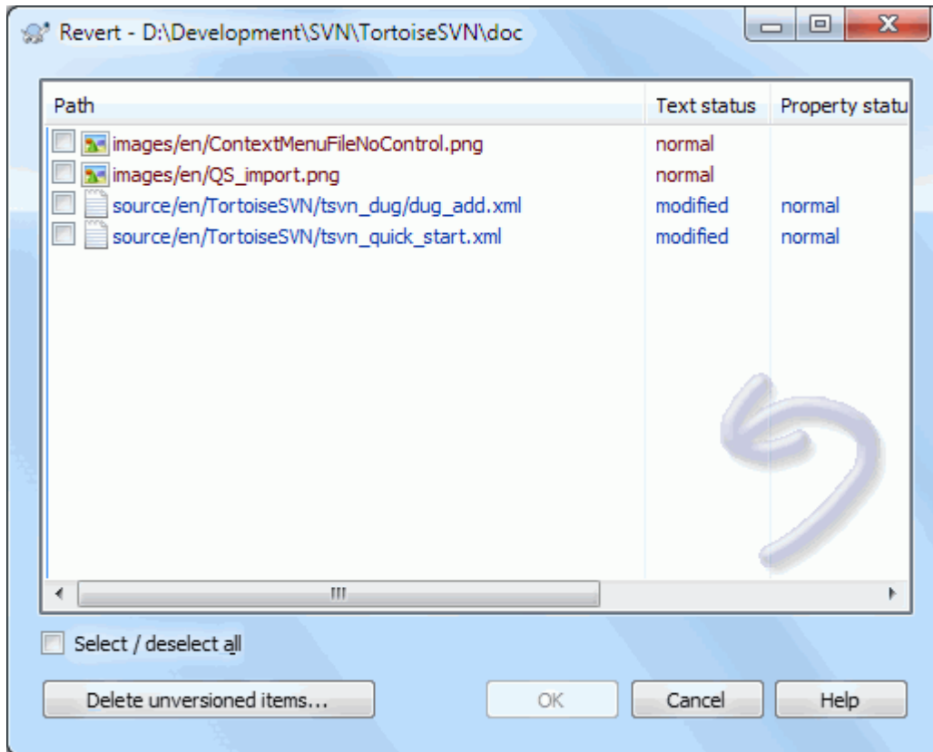
图 4.34. 恢复对话框
