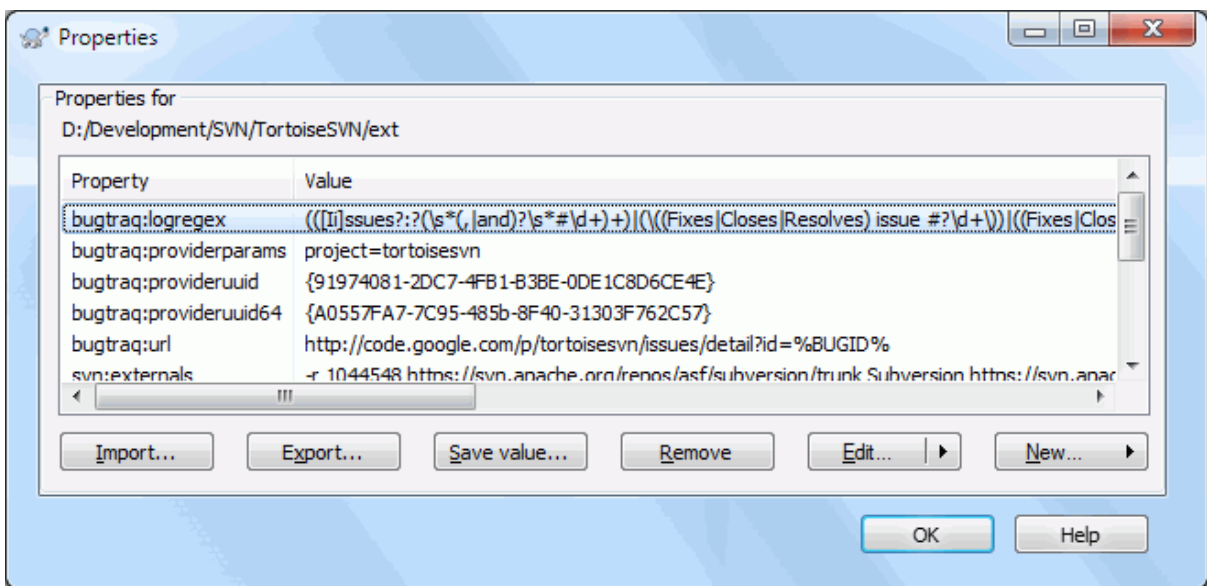
图 4. 36. Subversion 属性页
