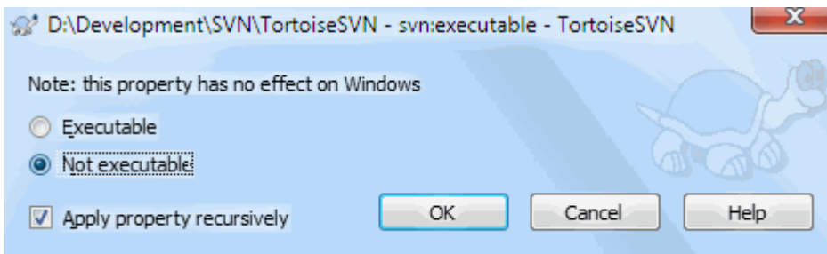
图 4.51. svn:executable 属性页
