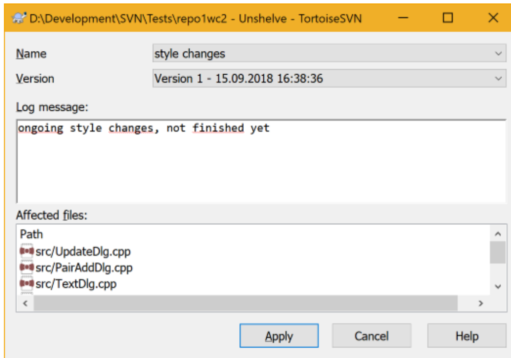
图 4.17. Unshelve dialog
