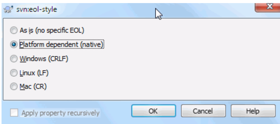
图 4.45. svn:eol-style 属性页
