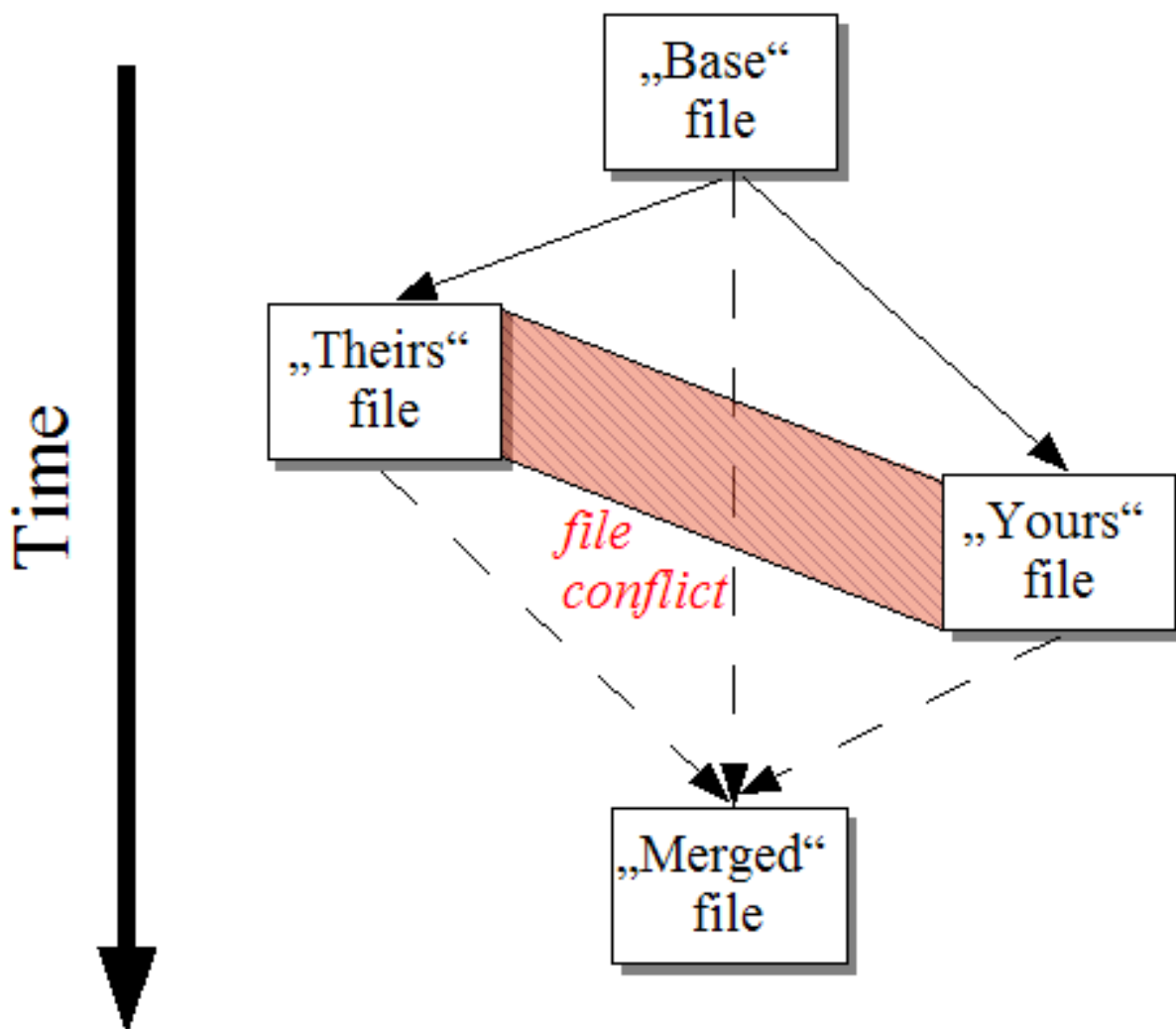
Afbeelding 1.1. Bestandsconflict
