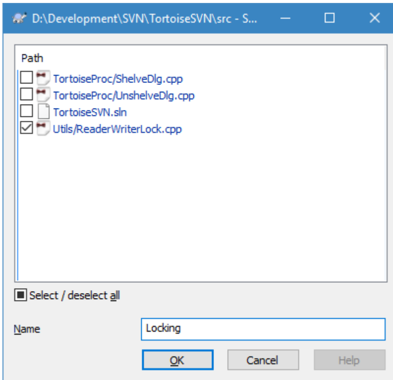
图 4.16. Shelve dialog
