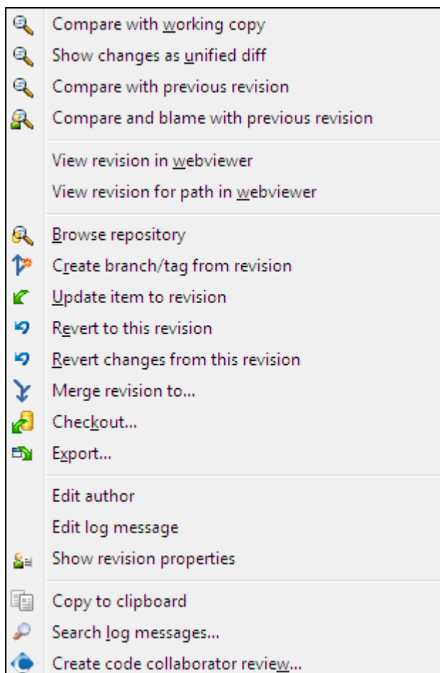
Obrázok 4.19. The Revision Log Dialog Top Pane with Context Menu
