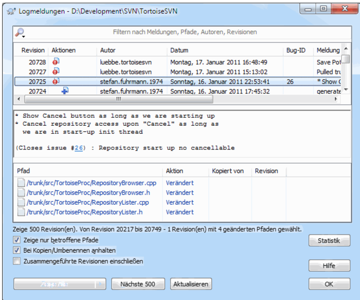
Abbildung 4.18. Der Log-Dialog
