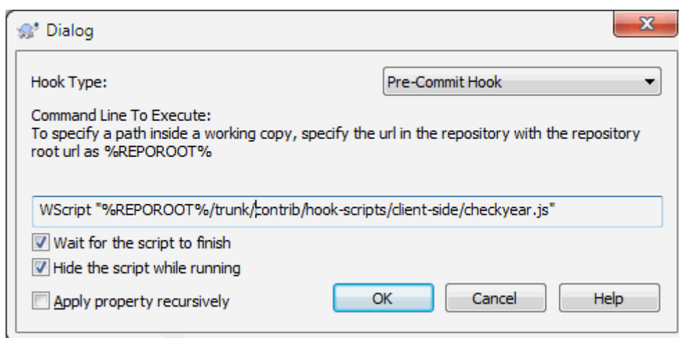
Obrázok 4.39. Property dialog for hook scripts
