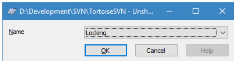
Obrázok 4.17. Unshelve dialog
