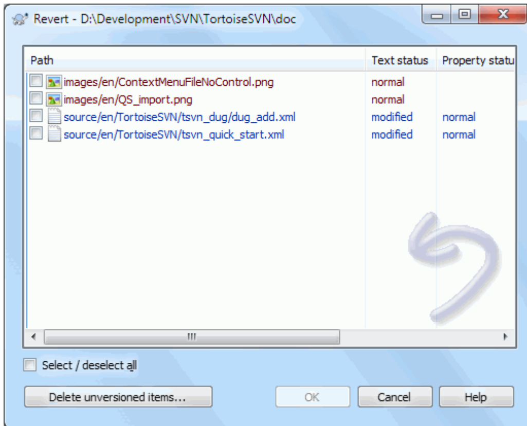
Obrázok 4.35. Dialóg vrátenia
