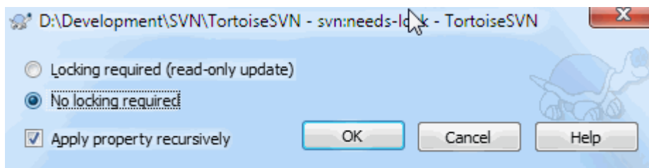
Slika 4.48. svn:traži-zaključavanje
