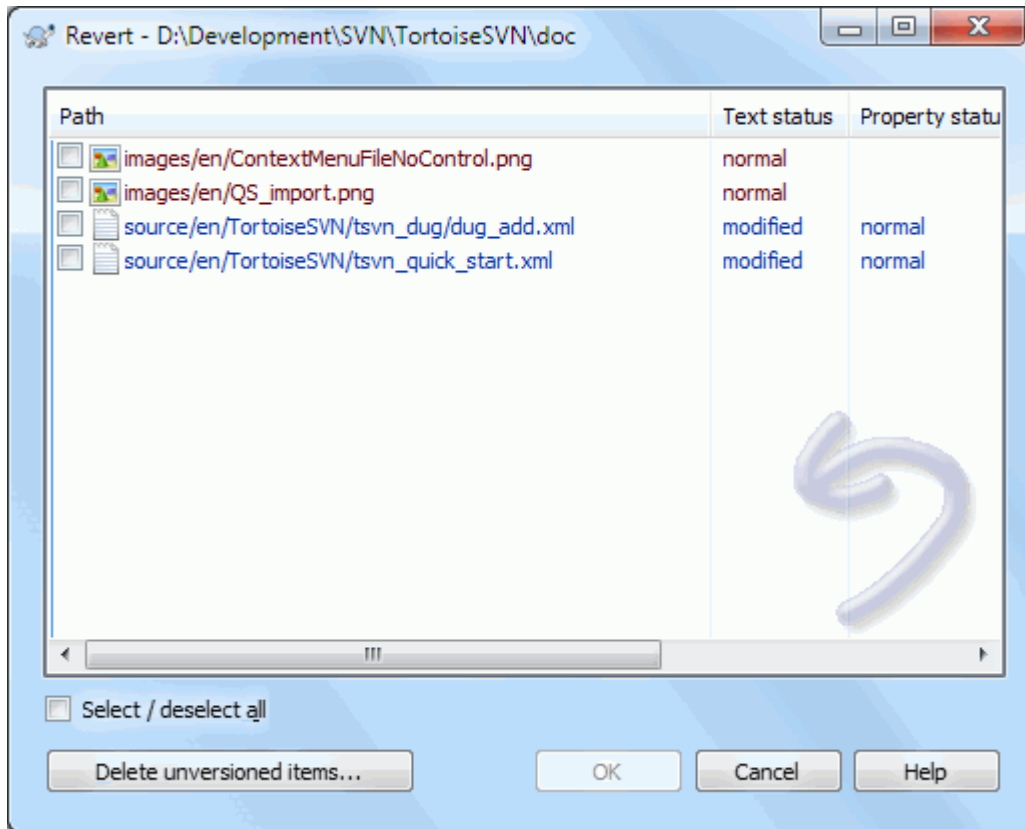
Slika 4.32. Vrați dijalog
