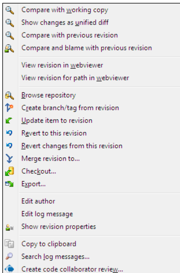
Slika 4.16. Gornji panel kontekstnog menija dnevnika dijaloga revizija
