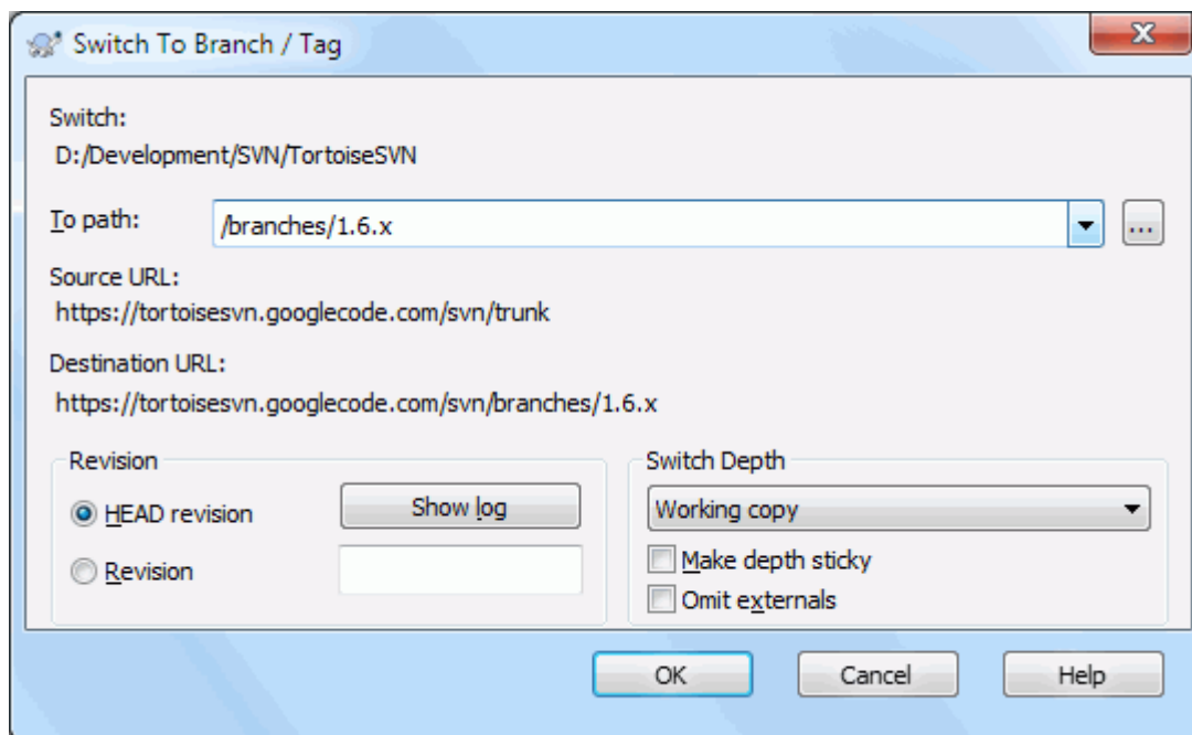
Slika 4.52. Prebaci dijalog
