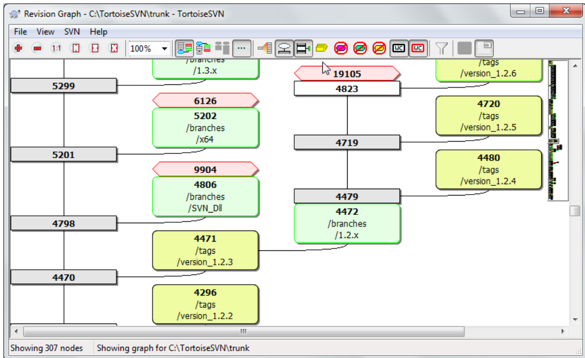
Slika 4.63. Revizioni graf
