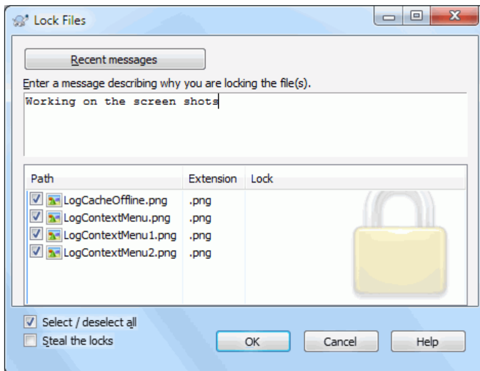
Slika 4.57. Dijalog zaključavanja
