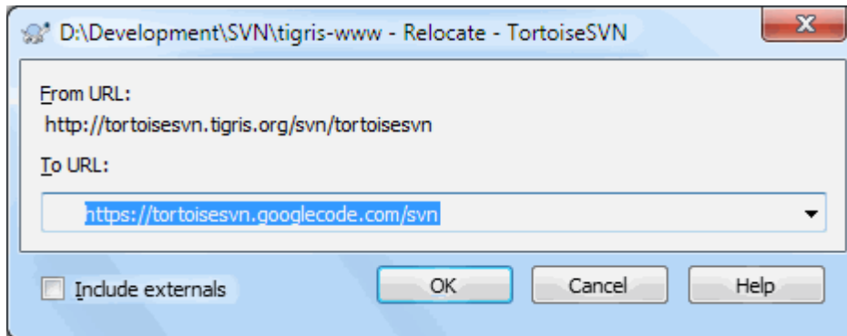
Slika 4.65. Relociranje dijaloga
