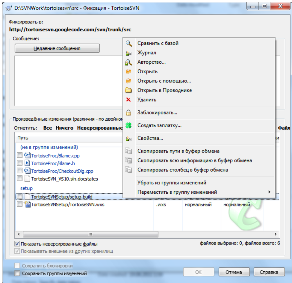
Рисунок 4.8. Диалог фиксации
