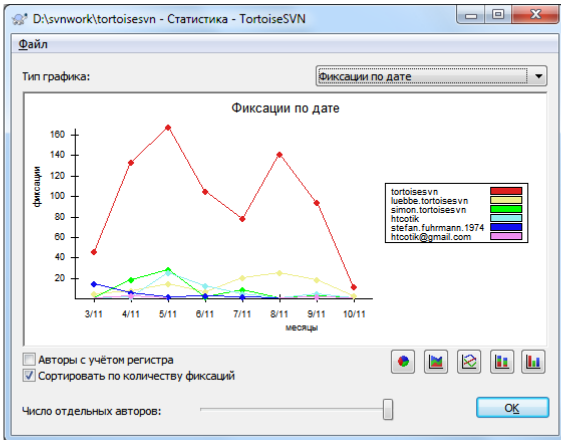
Рисунок 4.25. График Фиксации-по-датам
