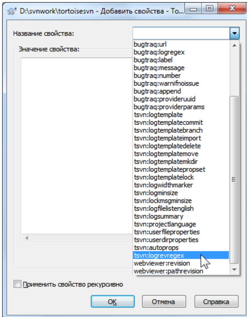
Рисунок 4.36. Добавление свойств
