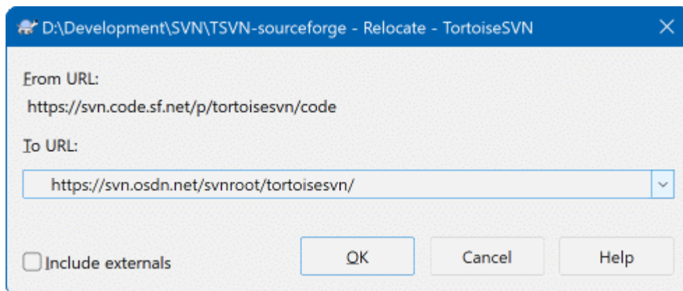
图 4.67. 重定位对话框
