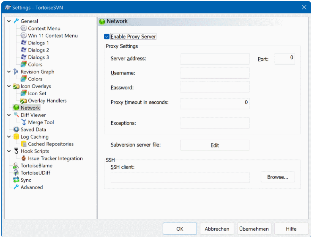
图 4.81. 设置对话框，网络设置页面
