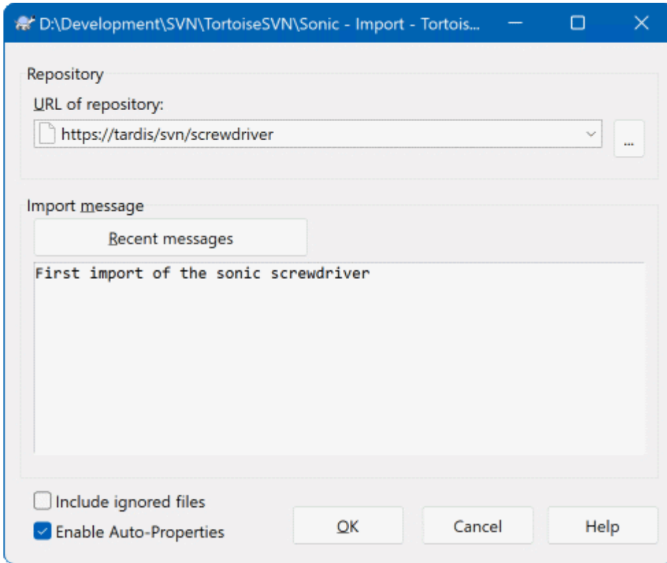
图 4.6. 导入对话框
