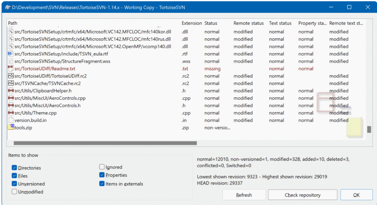
图 4.14. 检查修改
