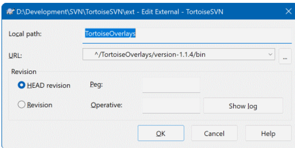
图 4.42. svn:externals 属性页
