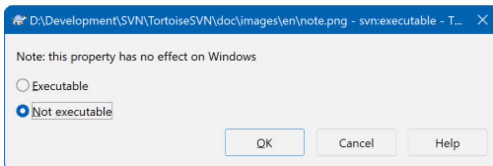
图 4.50. svn:executable 属性页
