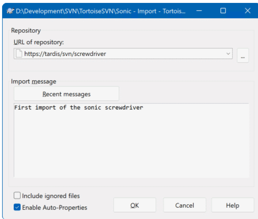
图 1.2. 导入对话框
