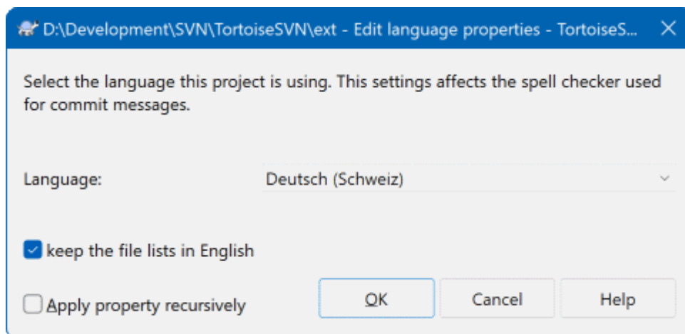
图 4. 47. 语言属性页
