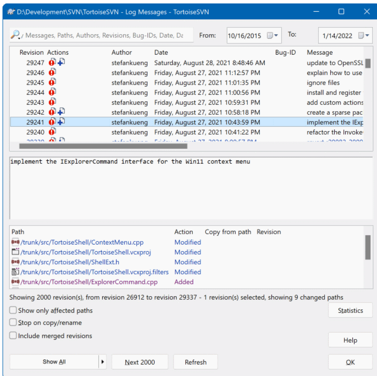
图 1.4. 日志对话框
