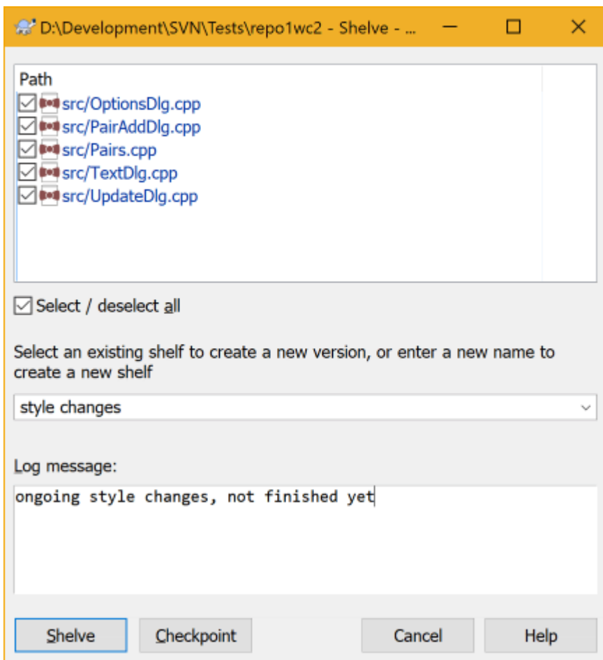
图 4.16. 搁置对话框
