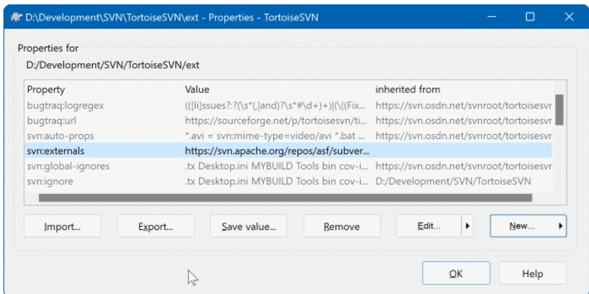
图 4. 35. Subversion 属性页
