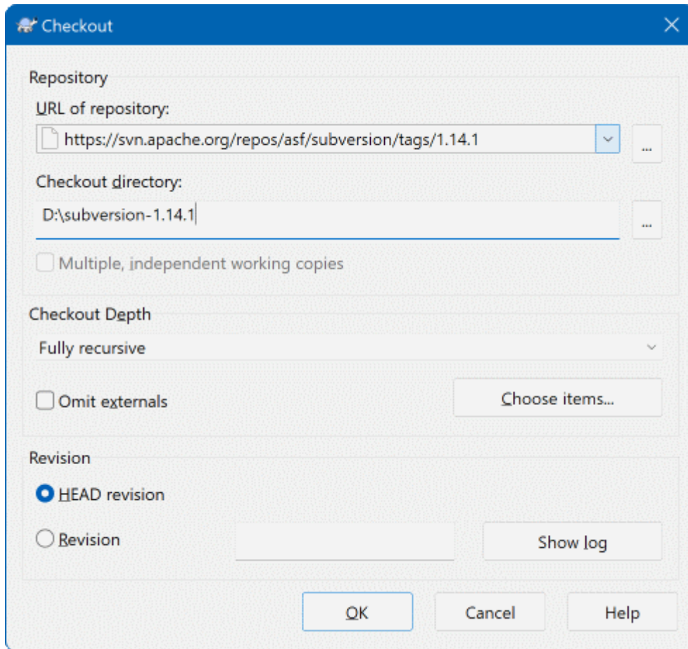
图 4.7. 检出对话框
