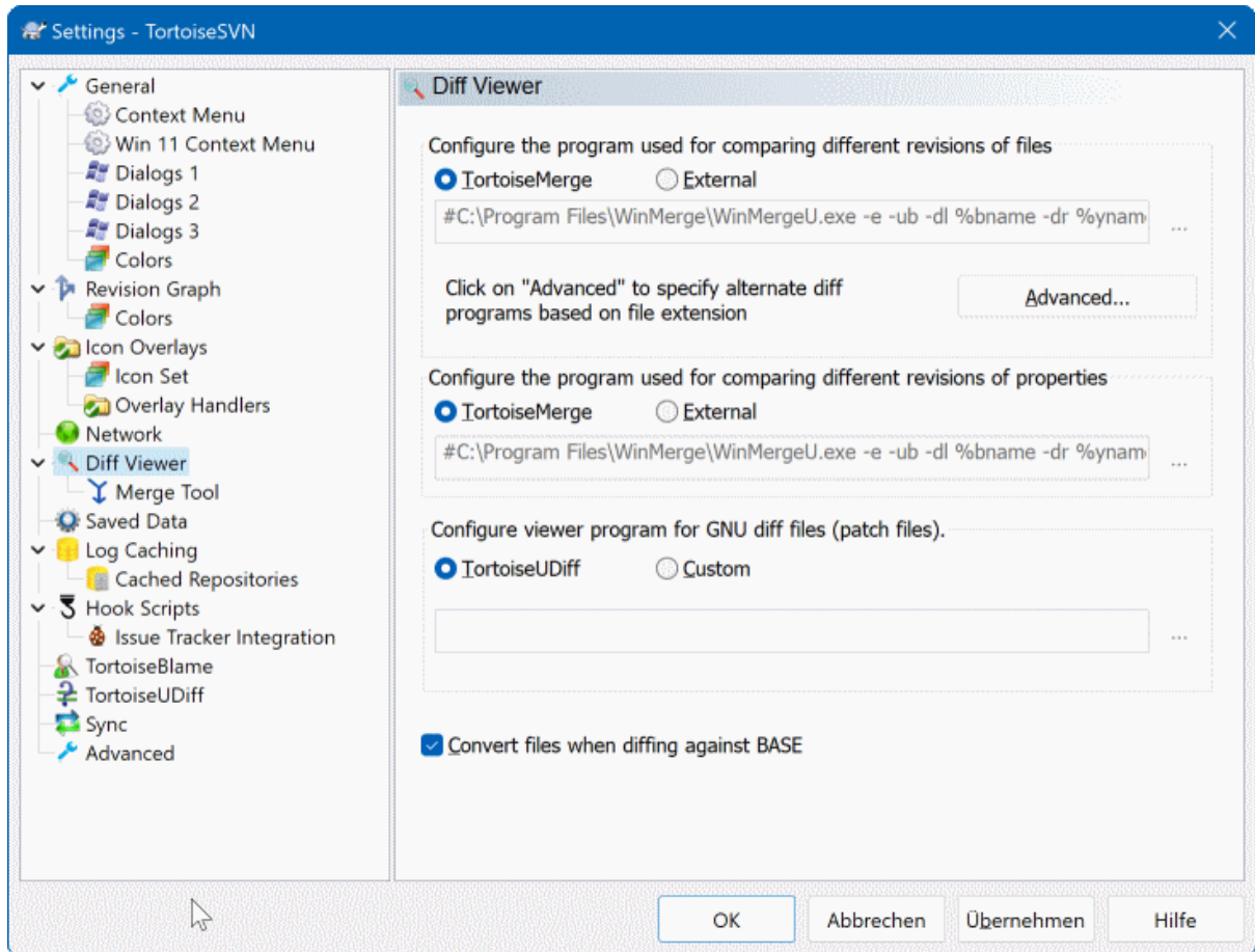
图 4. 82. 设置对话框，差异查看页面
