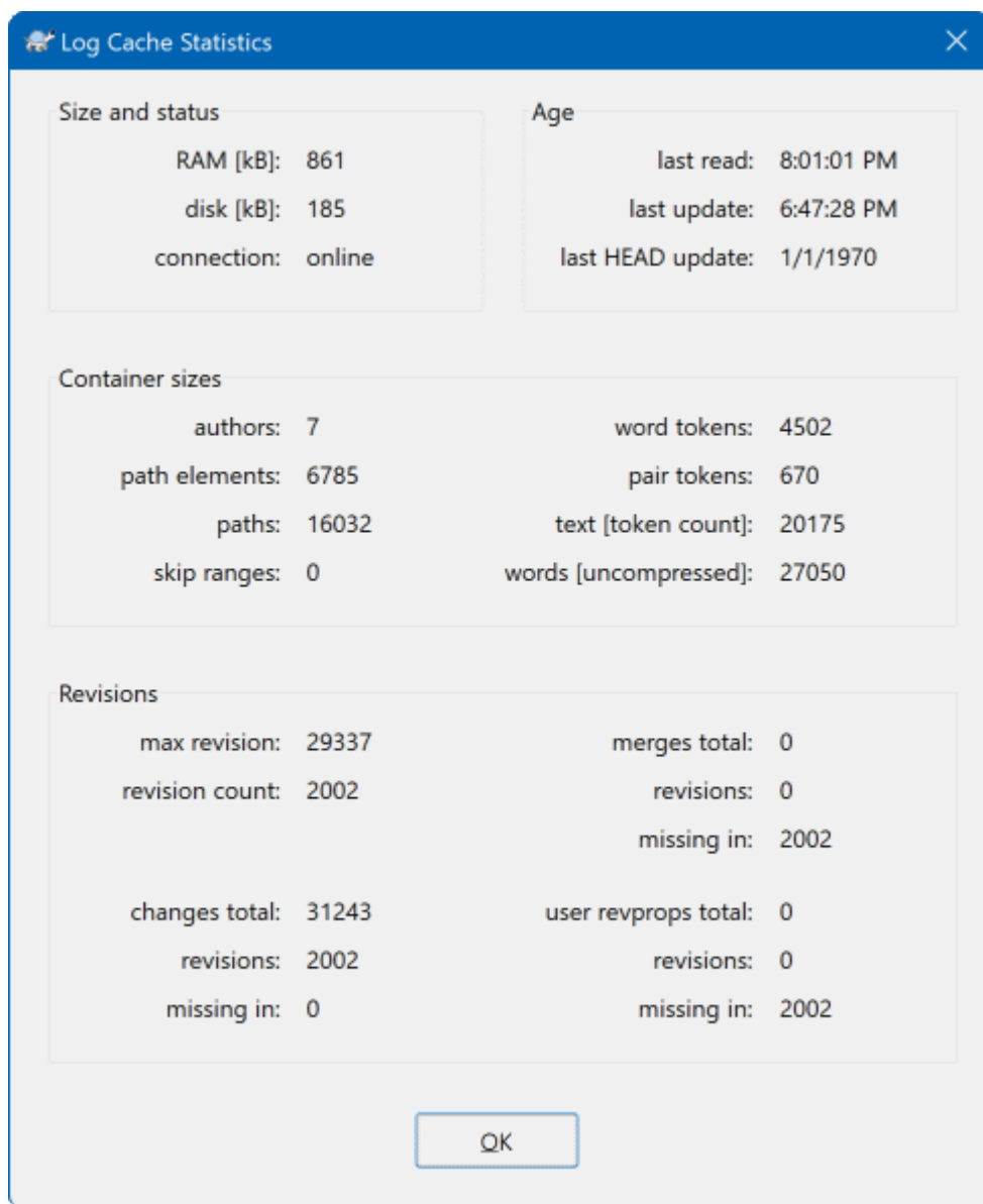
图 4.86. 设置对话框，日志缓存统计
