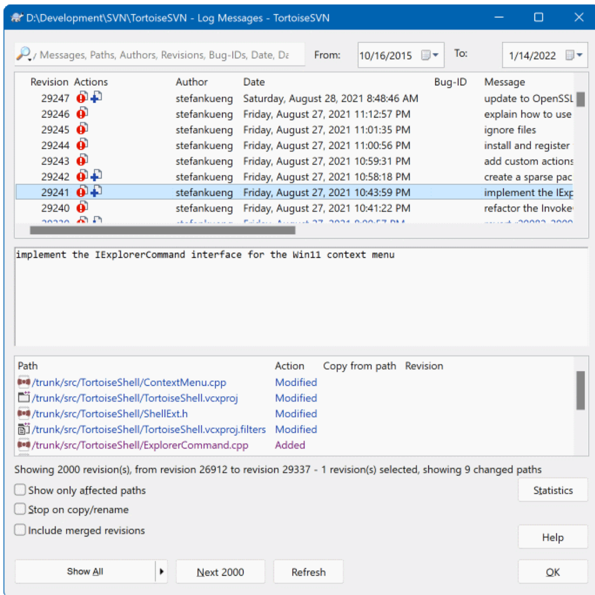
图 4.18. 版本日志对话框
