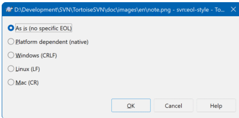
图 4.44. svn:eol-style 属性页
