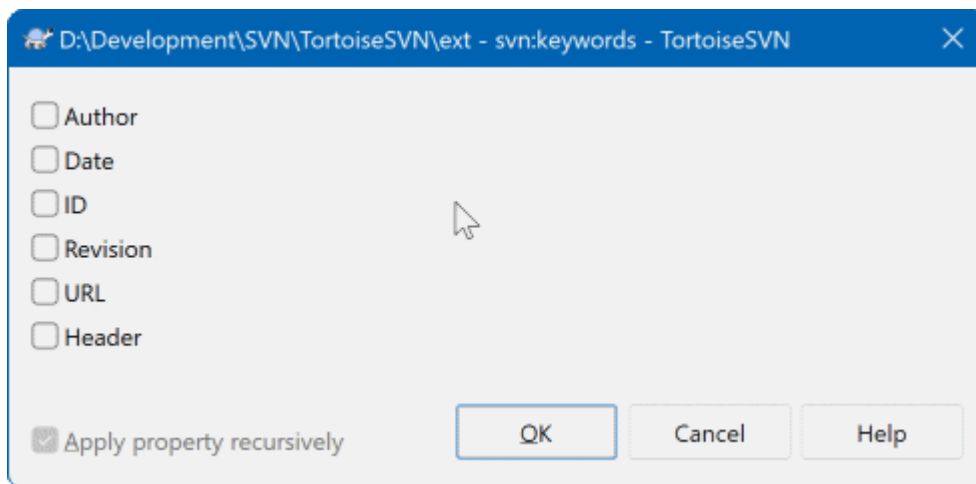
图 4.43. svn:keywords 属性页
