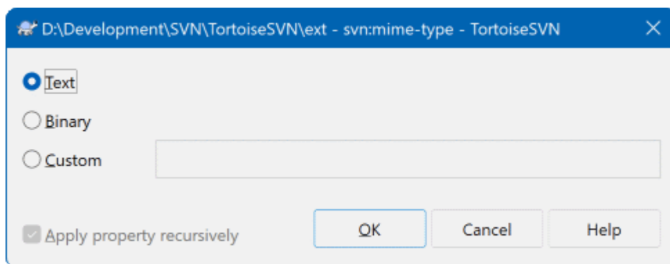
图 4.48. svn:mime-type 属性页
