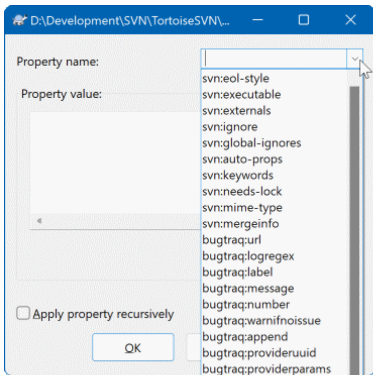
图 4.36. 增加属性
