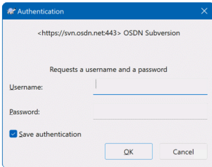
图 4.5. 认证对话框
