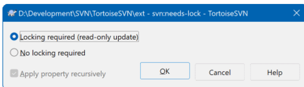
图 4.49. svn:needs-lock 属性页
