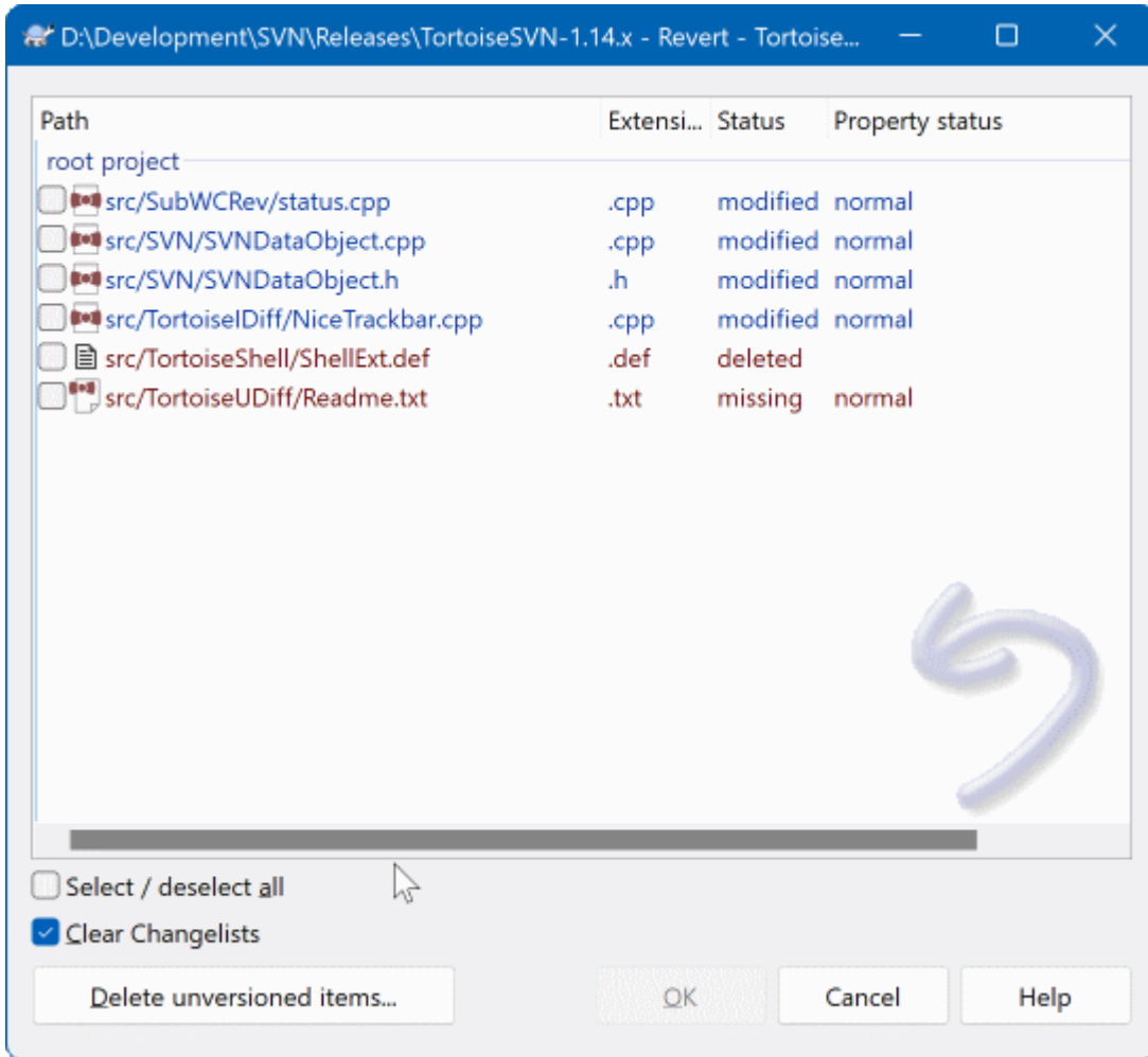
图 4.33. 恢复对话框
