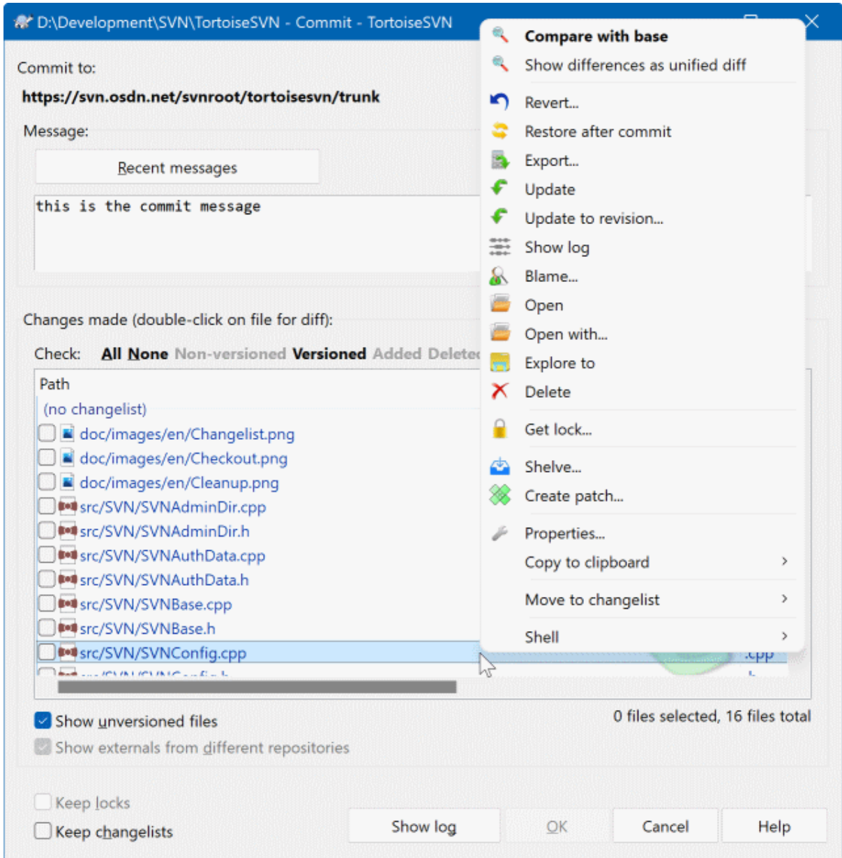
图 4.8. 提交对话框
