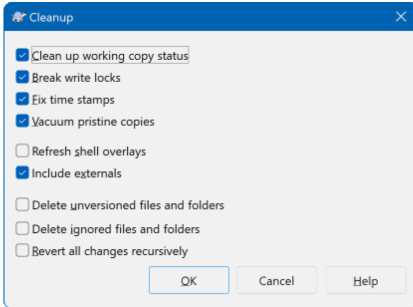
图 4.34. 清理对话框
