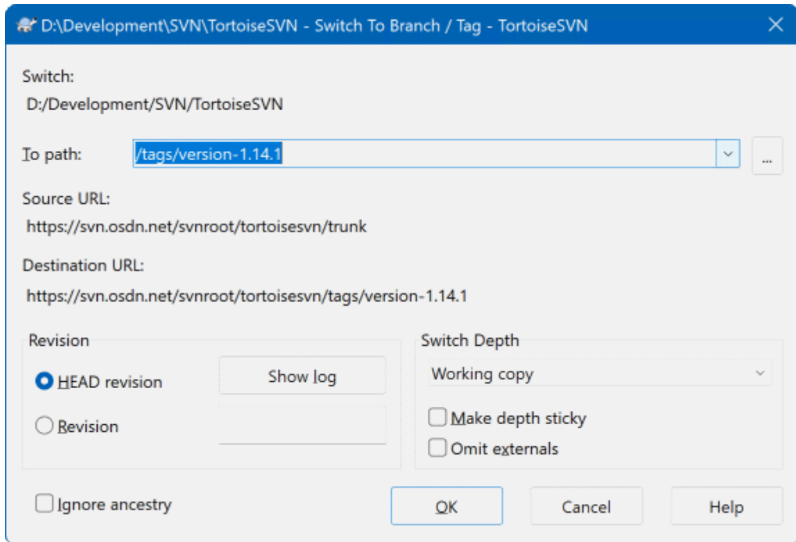
图 4.53. 切换对话框
