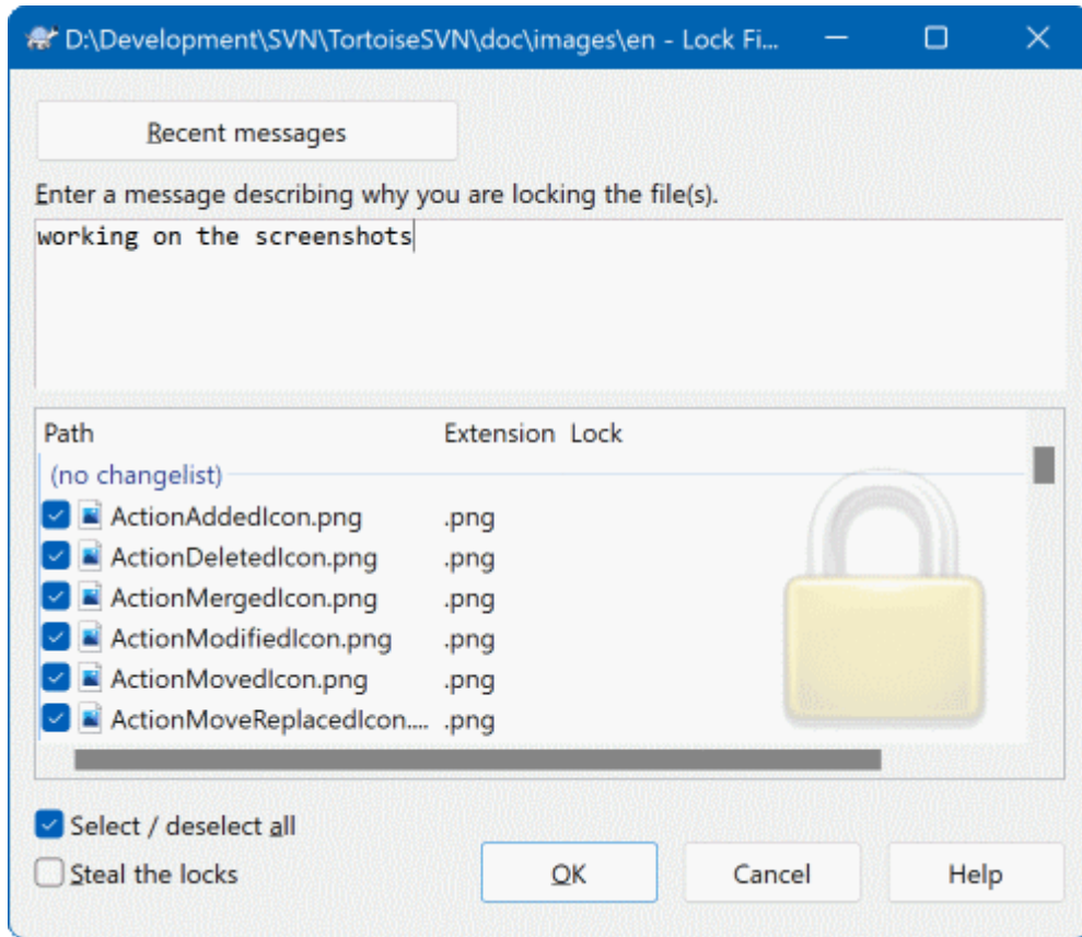
图 4.59. 锁定对话框
