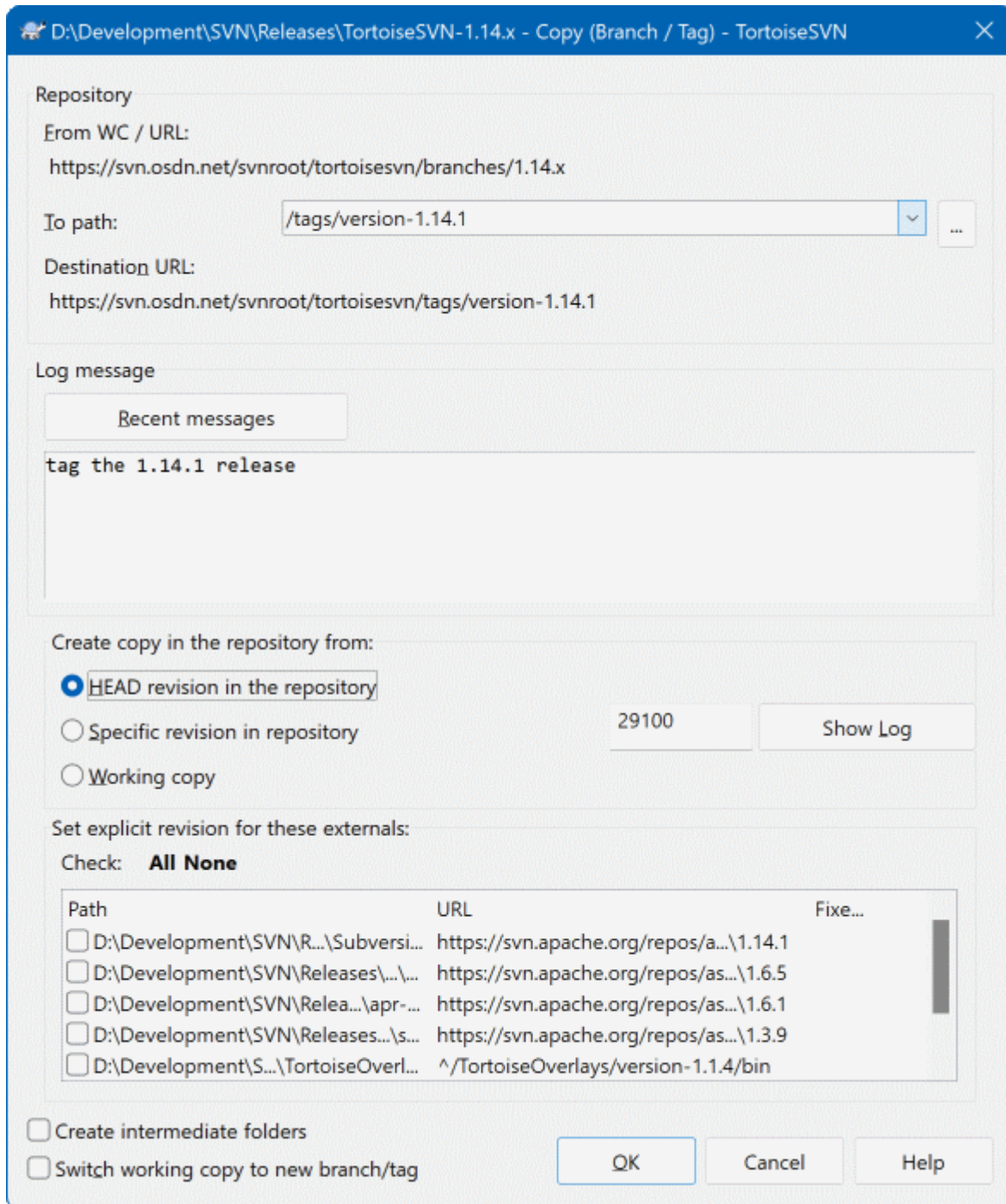
图 4.52. 分支/标记对话框
