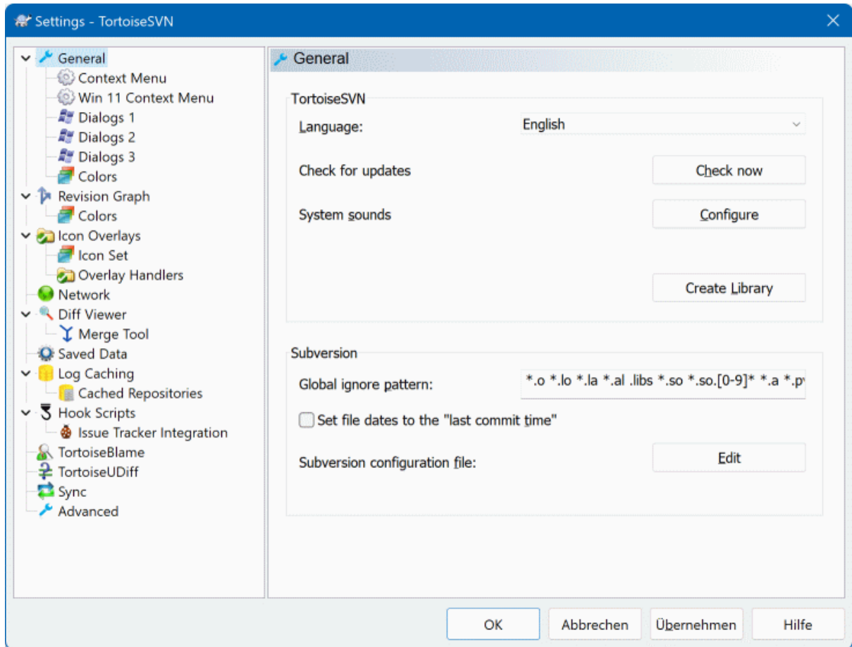
图 4. 70. 设置对话框，常规设置页面
