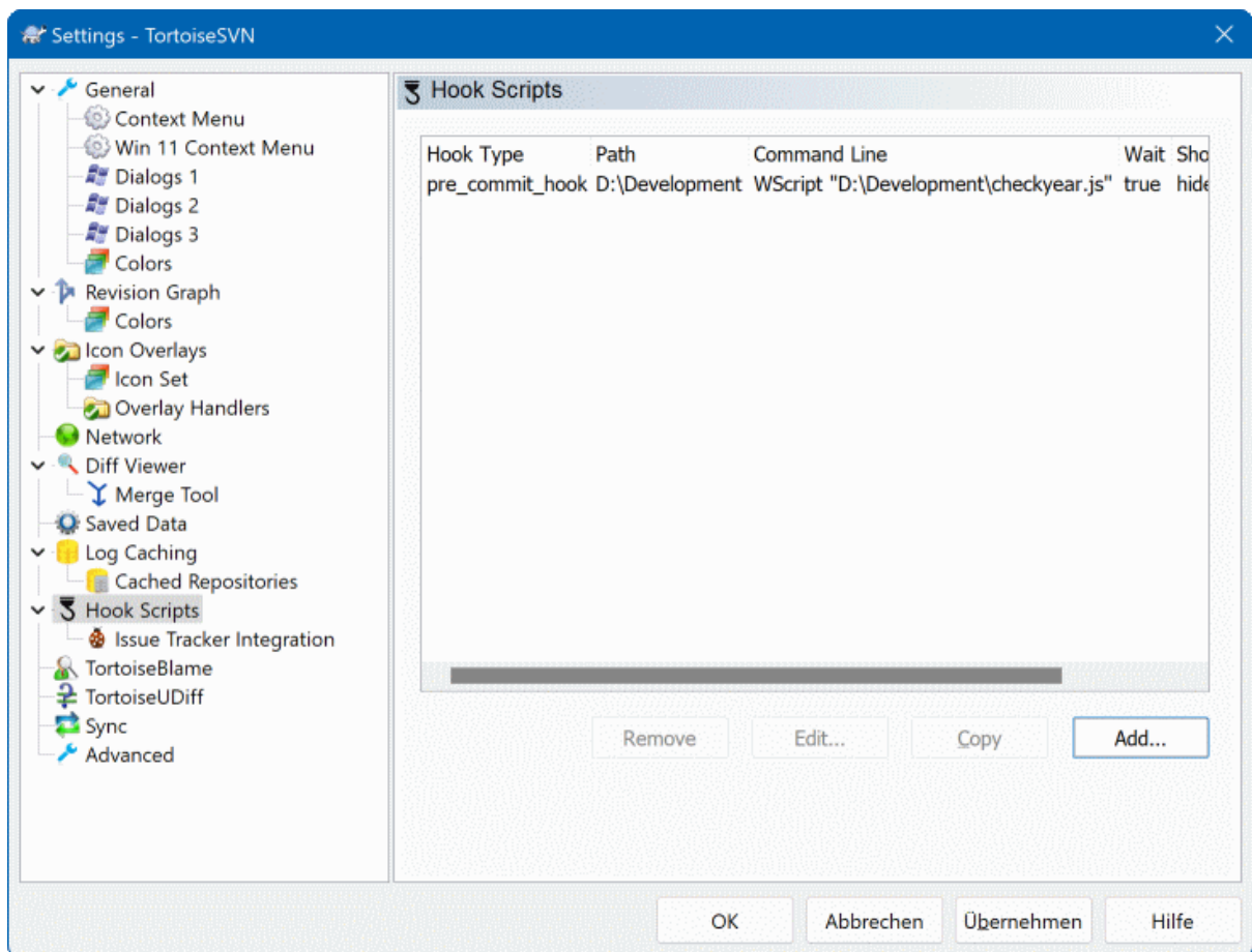
图 4. 87. 设置对话框，钩子脚本页
