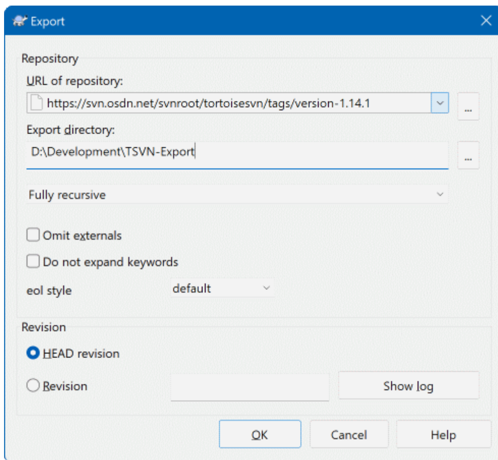
图 4.66. 从 URL 导出对话框
