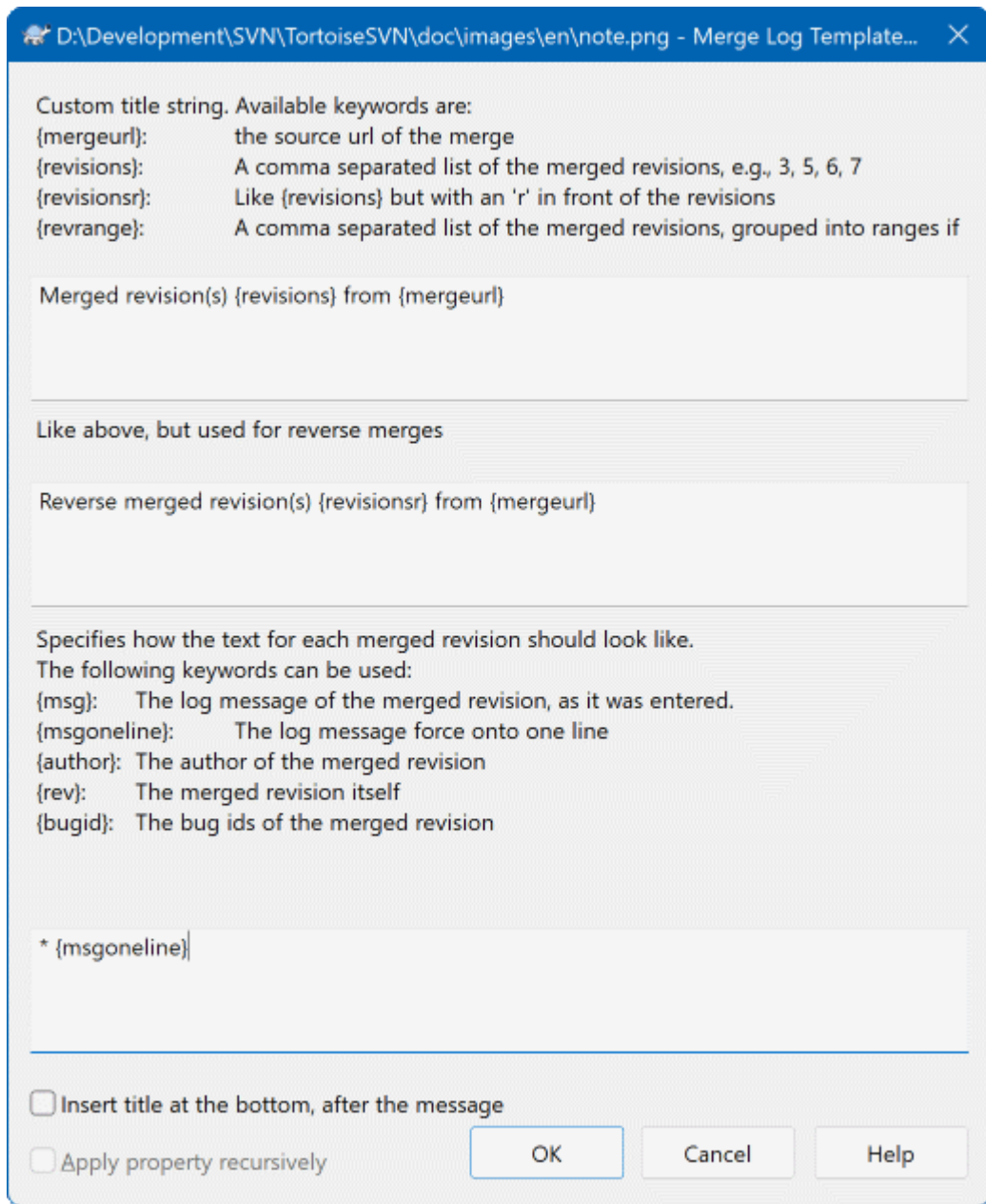
图 4.51. 合并日志信息模板属性对话框
