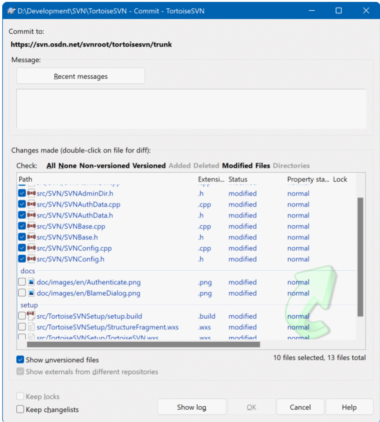
图 4.15. 带有修改列表的提交对话框
