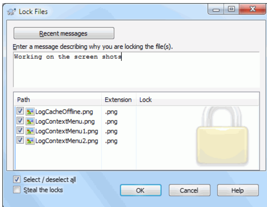
图 4.59. 锁定对话框
