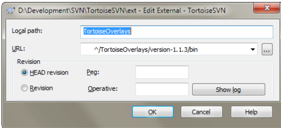
图 4.42. svn:externals 属性页
