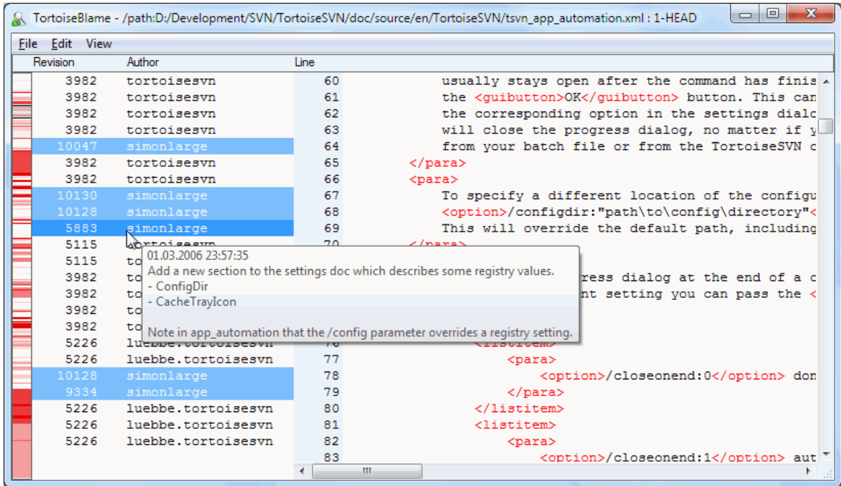
图 4.63. TortoiseBlame
