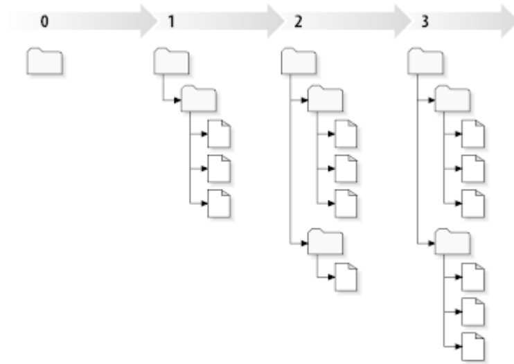
図2.7 リポジトリ
