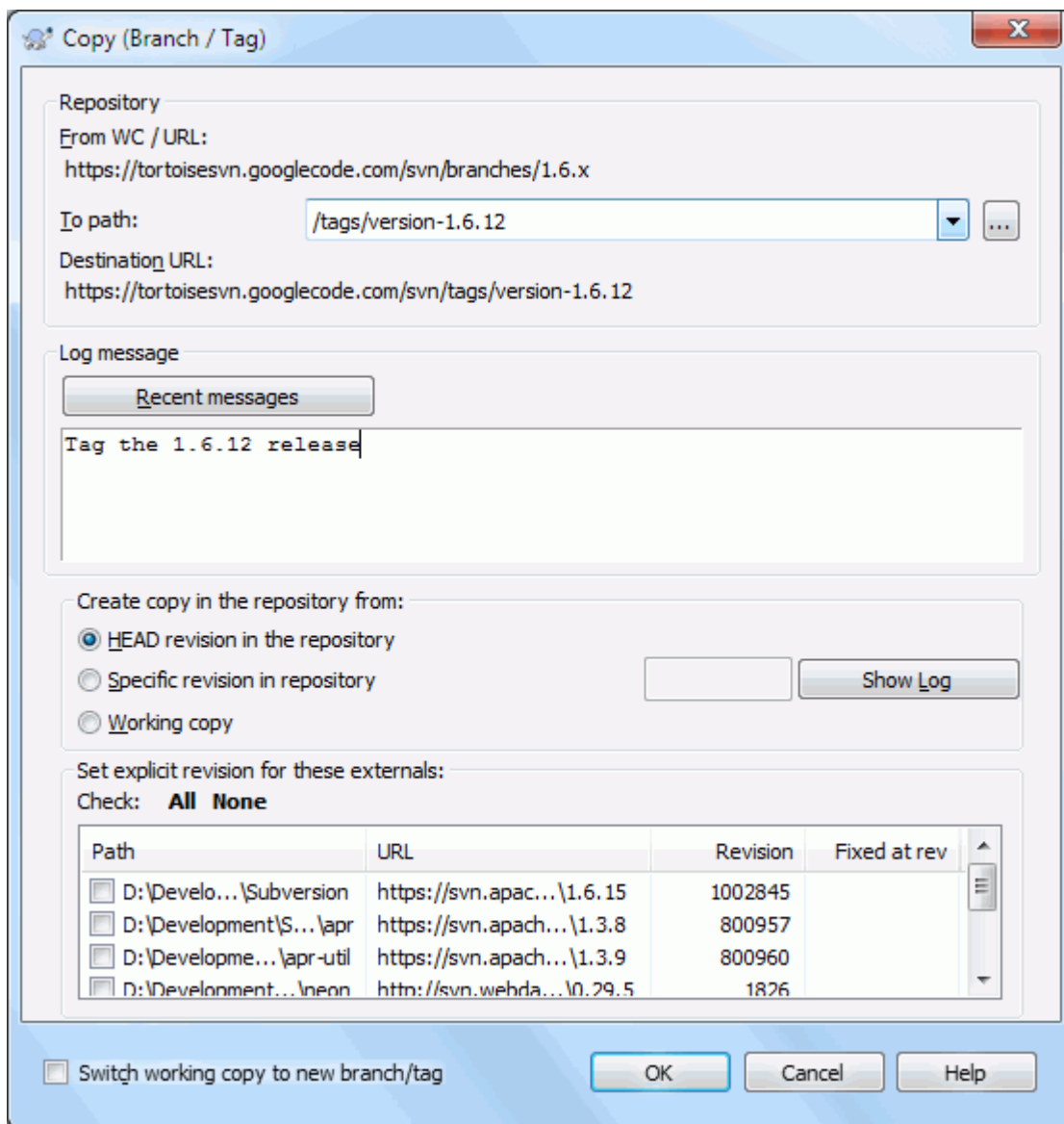
图 4.52. 分支/标记对话框
