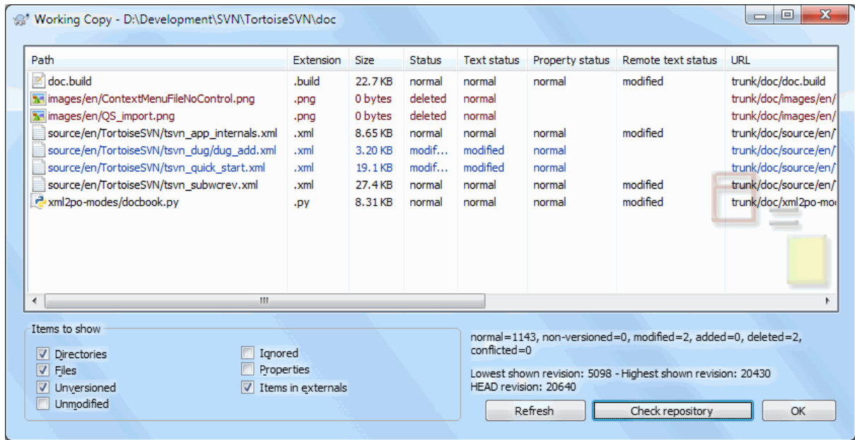
图 4. 60. 检查修改对话框
