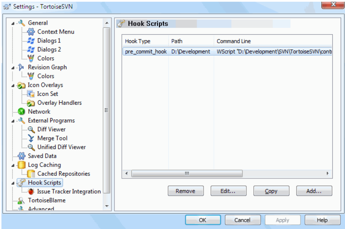
图 4.87. 设置对话框，钩子脚本页
