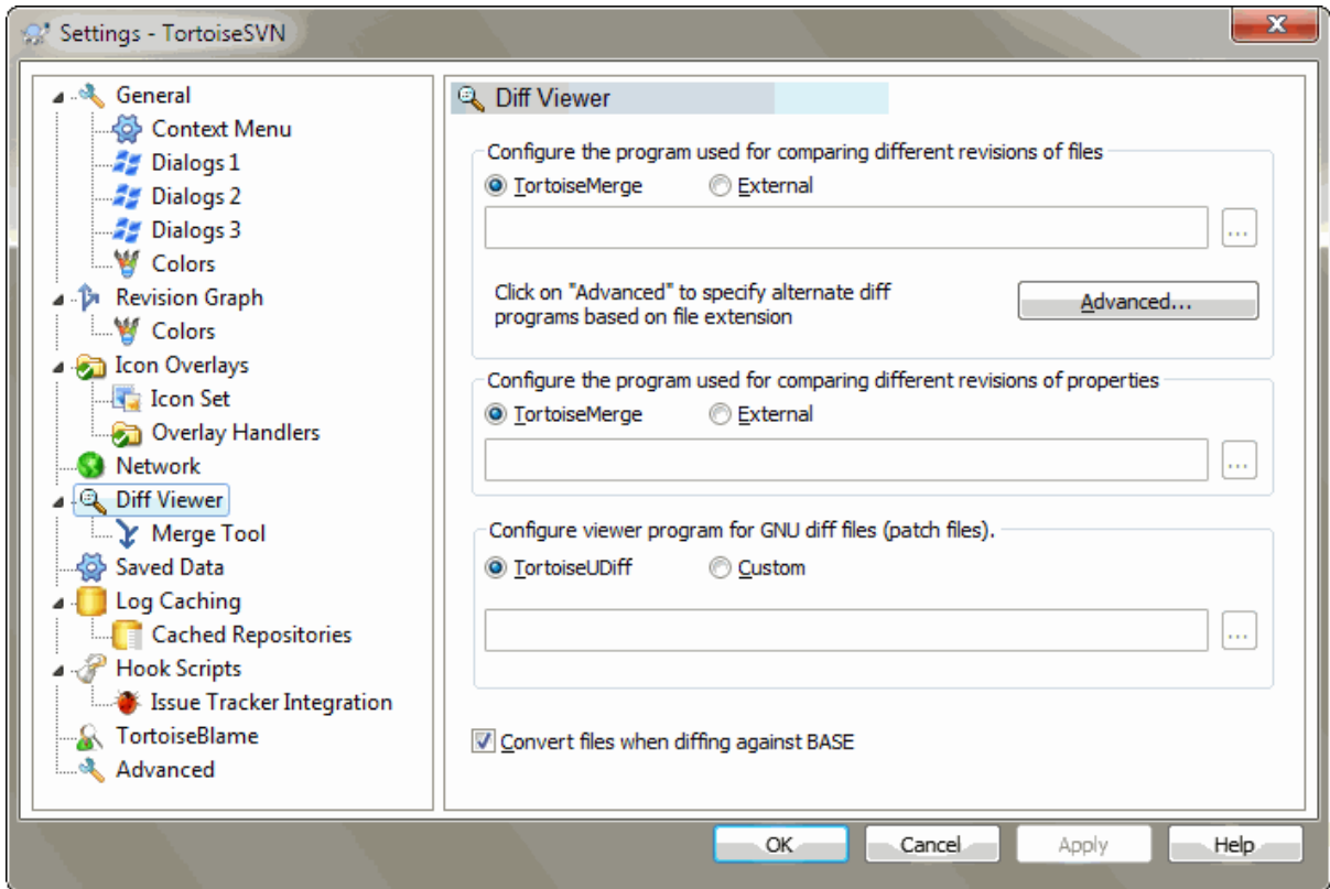
图 4. 82. 设置对话框，差异查看页面
