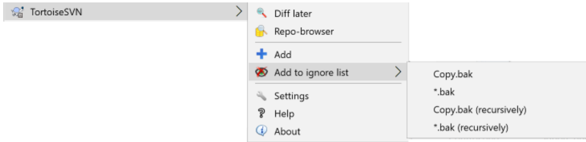
图 4.30. 未受版本控制的文件之资源管理器上下文菜单
