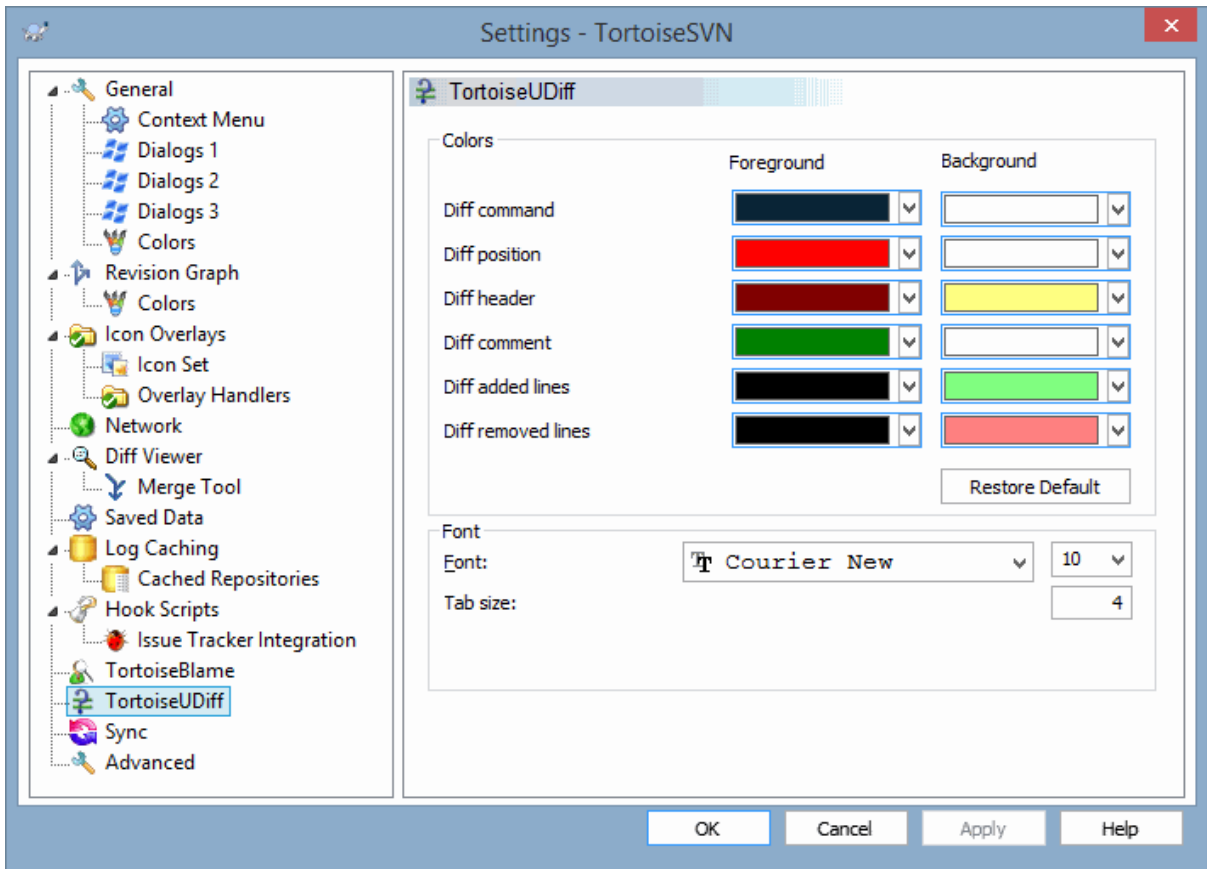
图 4.91. 设置对话框, TortoiseUDiff 页面
