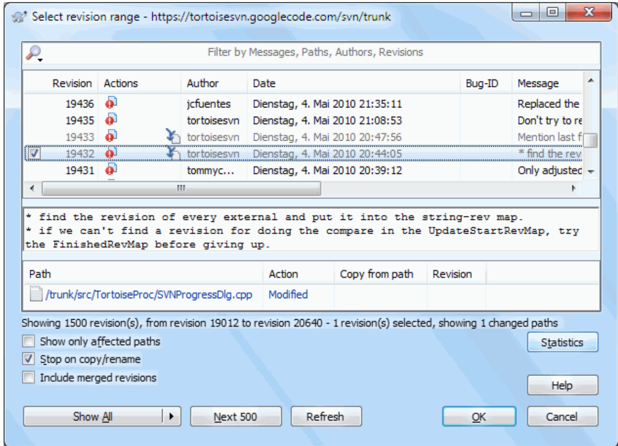
图 4. 23. 日志对话框显示合并跟踪版本
