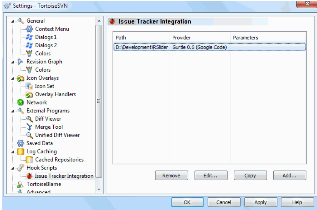
图 4.89. 设置对话框, 问题跟踪集成页
