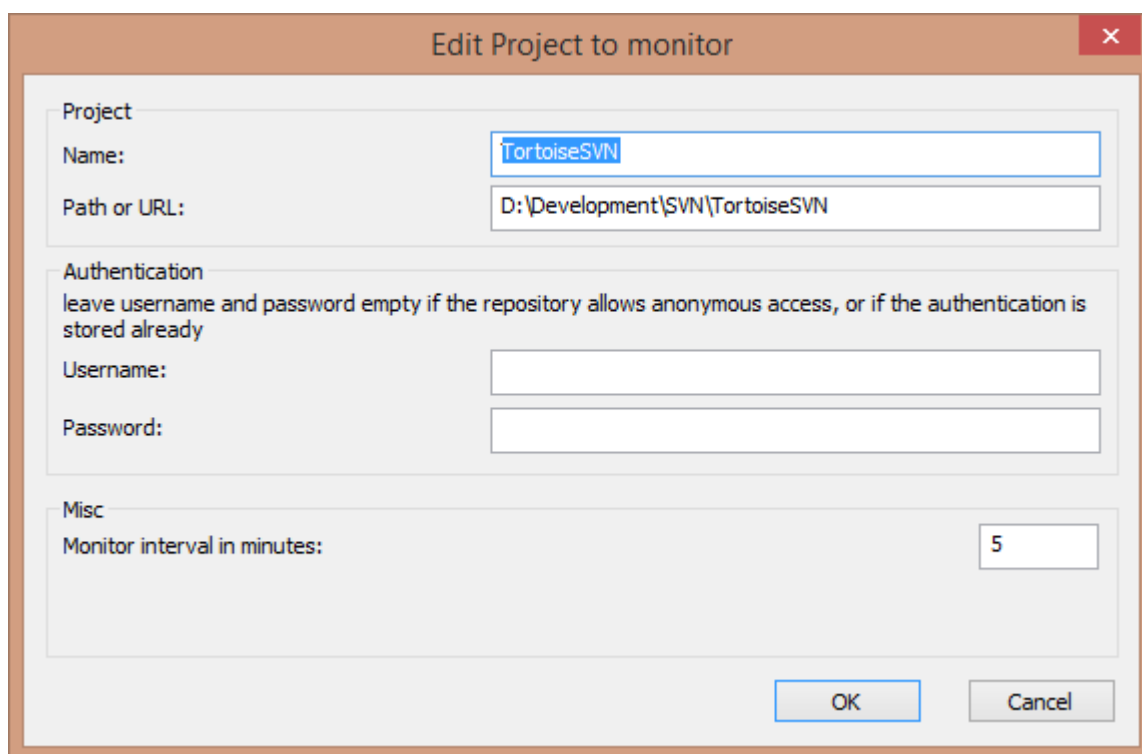
图 5.1. 项目监视器的编辑项目对话框
