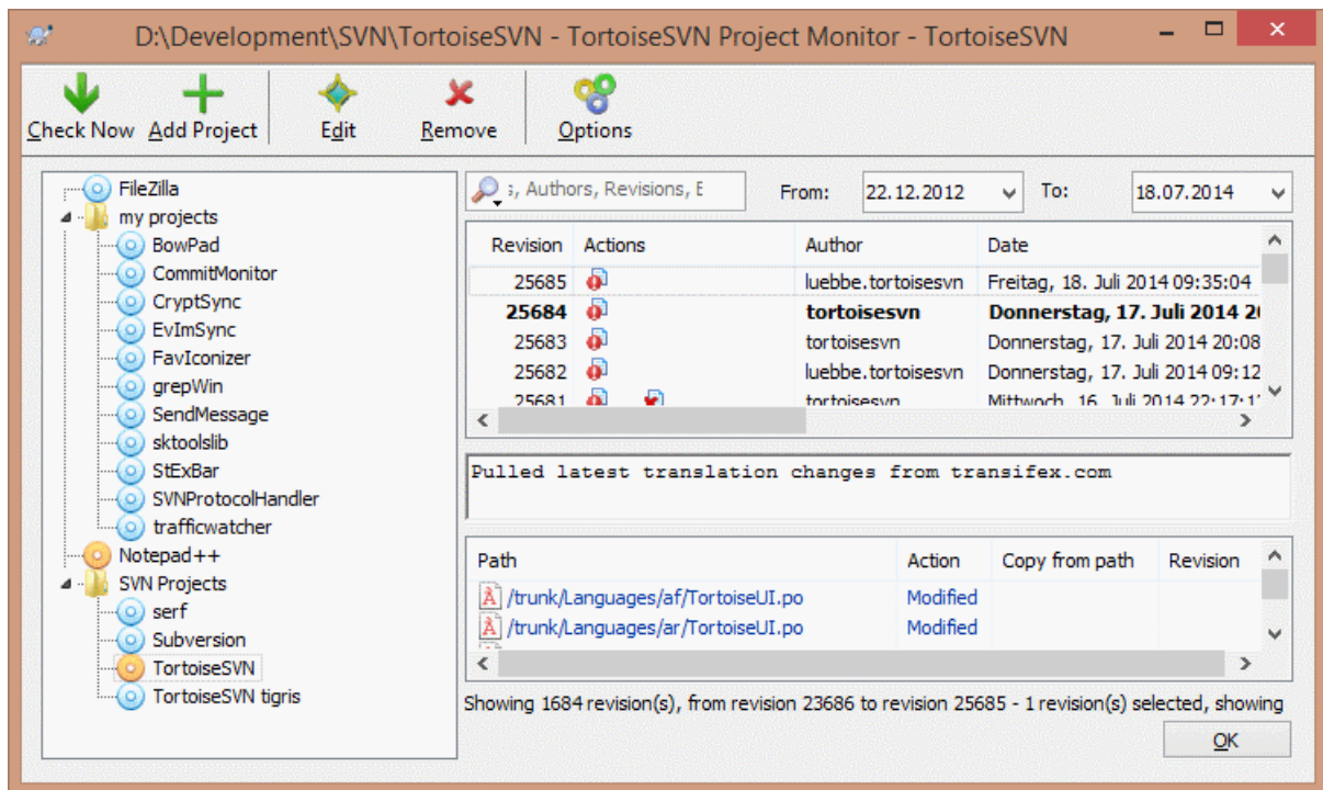
图 5.2. 项目监视器的主对话框
