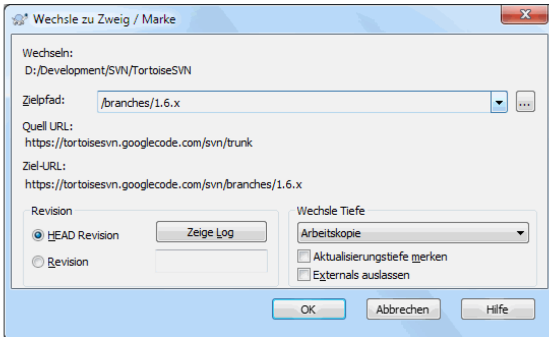
Abbildung 4.52. Der Wechseln-Zu-Dialog
