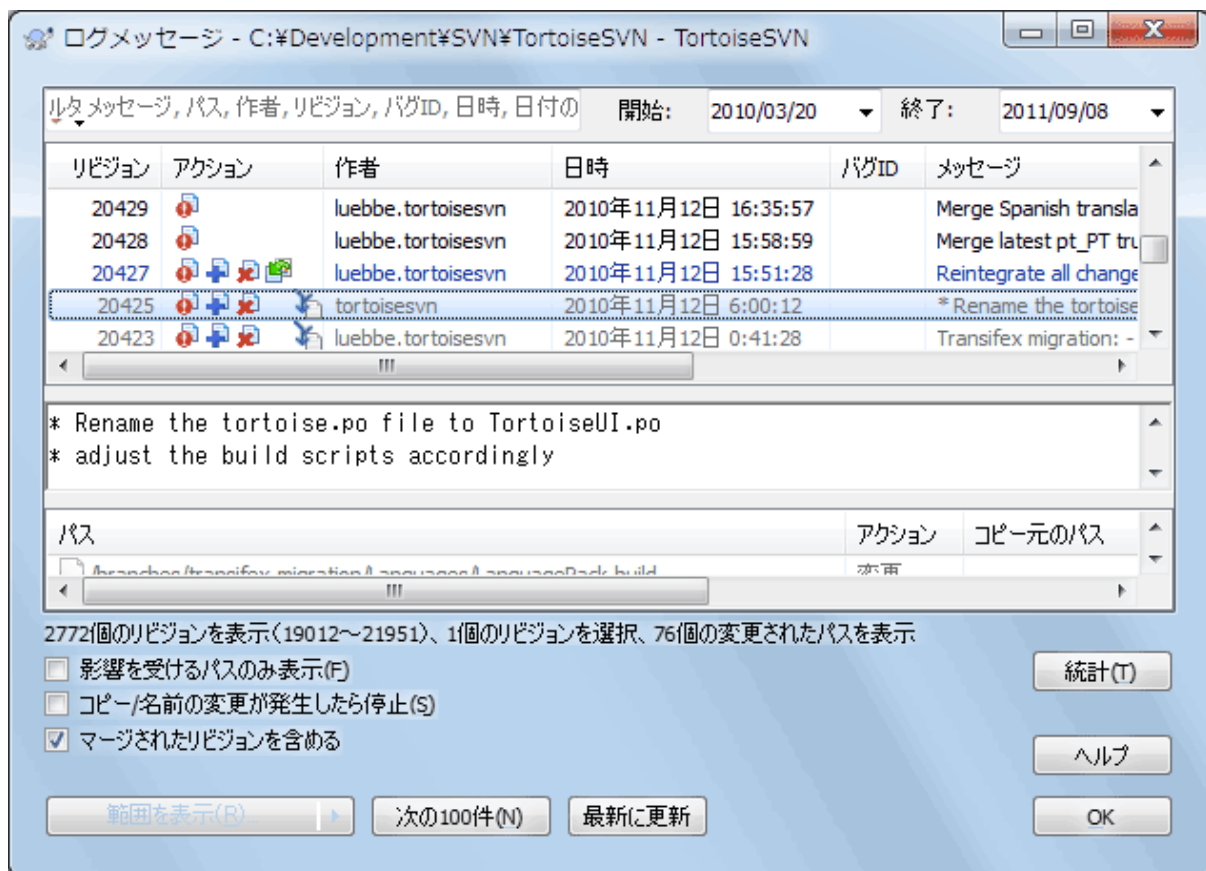
図4.24 マージ追跡リビジョンを表示したログダイアログ
