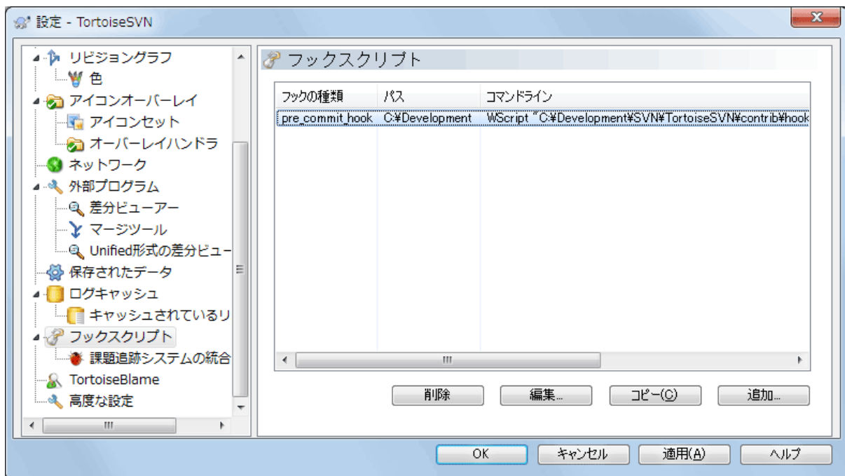
図4.89 設定ダイアログの「フックスクリプト」ページ
