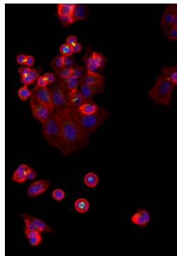
ImgFITC
